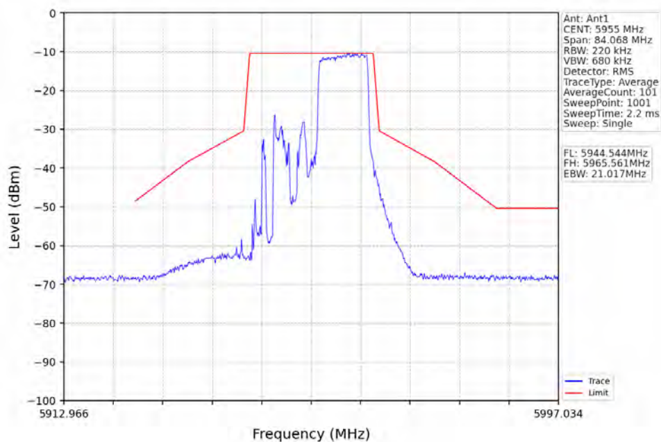
802.11ax(HEW20)_LCH_5955MHz_RU242_Left_Ant1_NTNV
