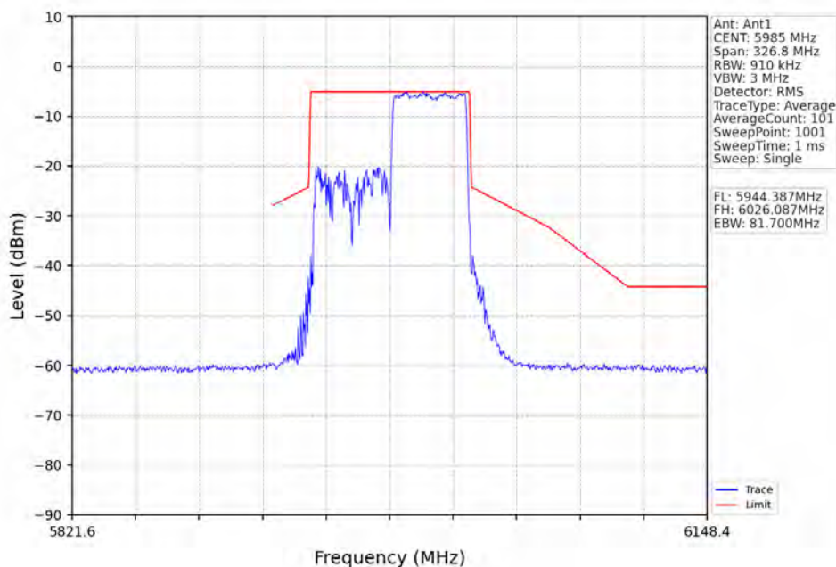
802.11ax(HEW80)_LCH_5985MHz_RU484_Right_Ant1_NTNV
