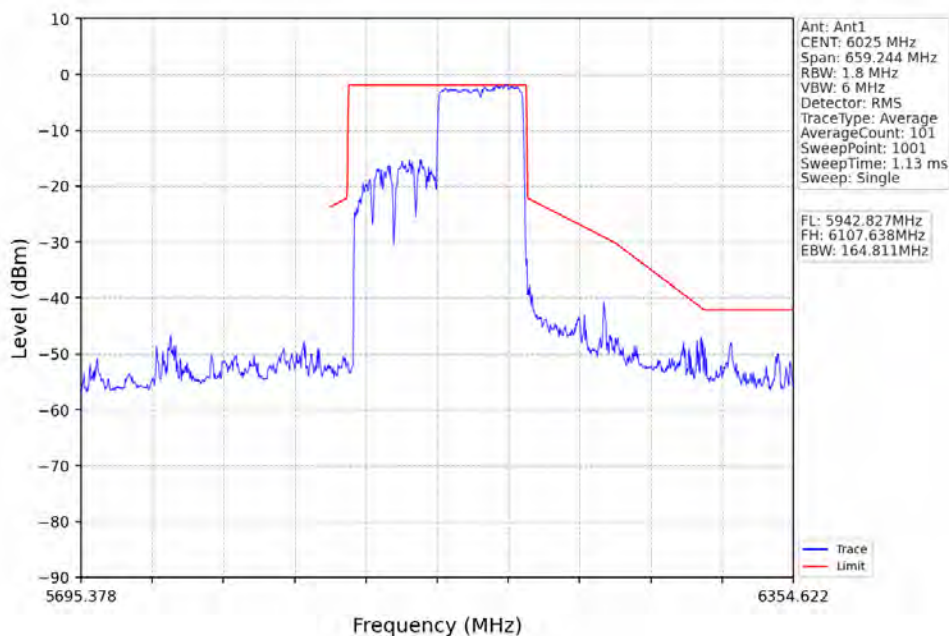
802.11ax(HEW160)_LCH_6025MHz_RU996_Left_Ant1_NTNV
