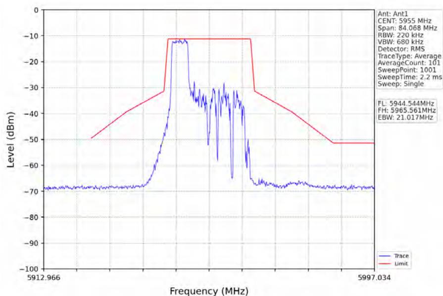
802.11ax(HEW20)_LCH_5955MHz_RU52_Right_Ant1_NTNV
