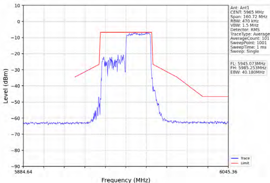
802.11ax(HEW40)_LCH_5965MHz_RU484_Left_Ant1_NTNV
