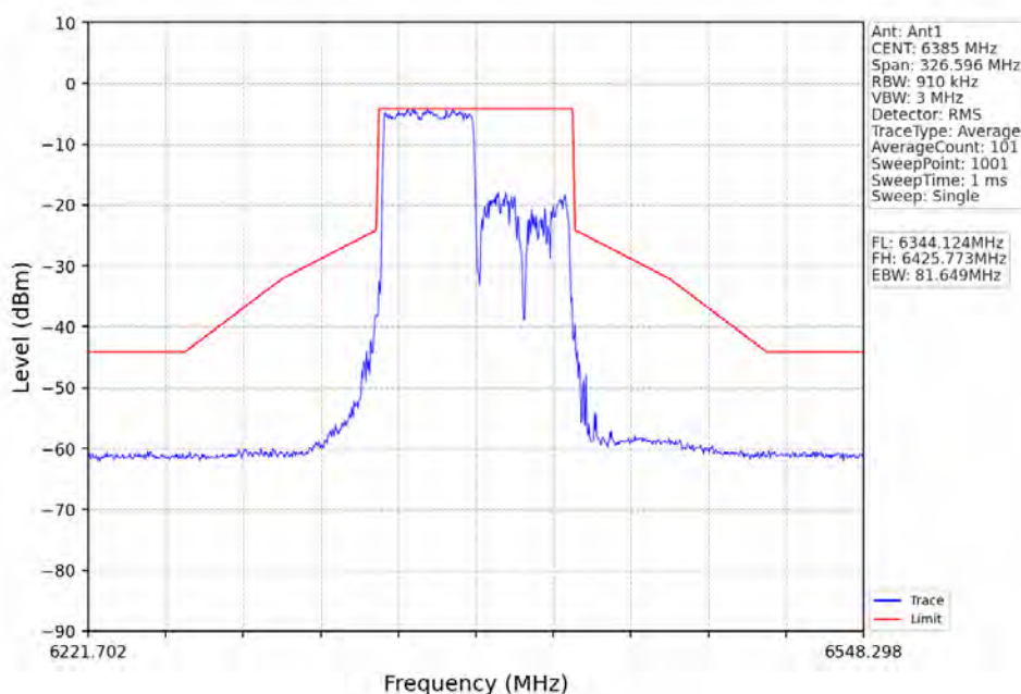
802.11ax(HEW80)_HCH_6385MHz_RU484_Right_Ant1_NTNV
