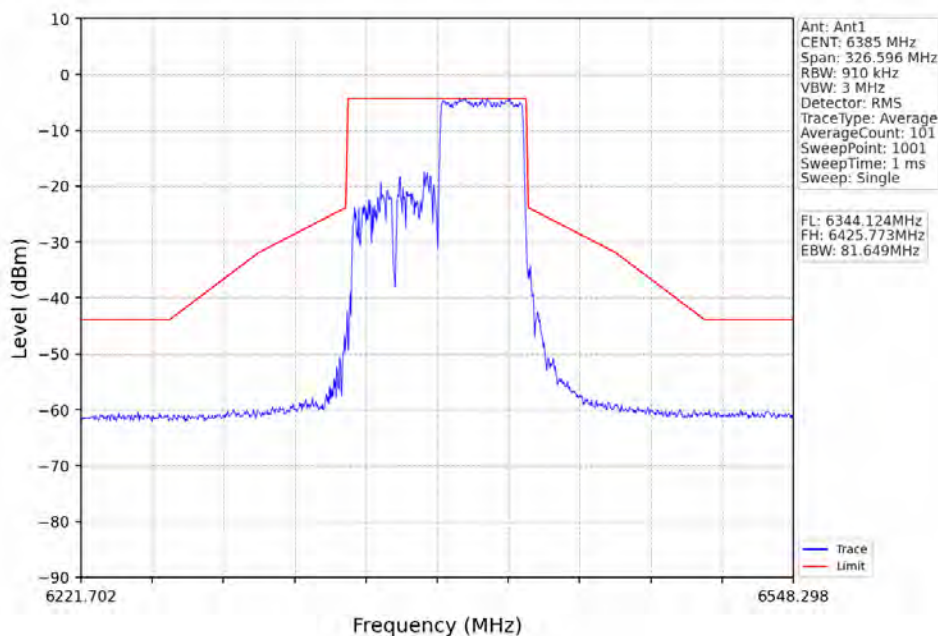
802.11ax(HEW80)_HCH_6385MHz_RU484_Right_Ant1_NTNV
