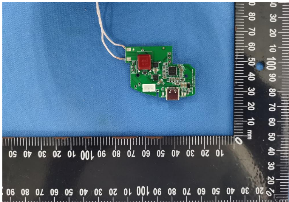
EUT Photo (16)
