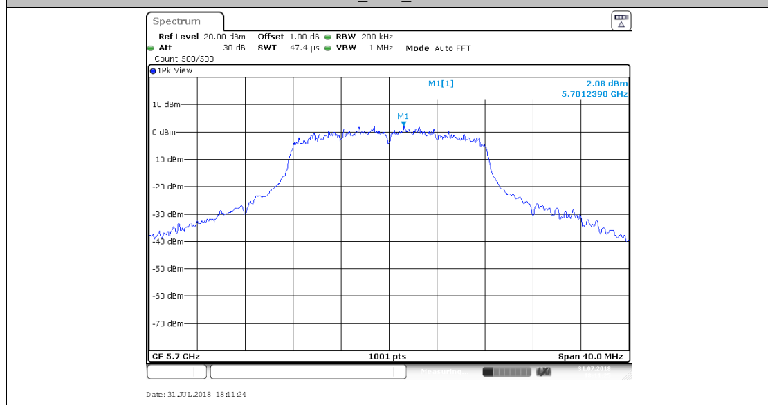
11A_Ant1_5700
