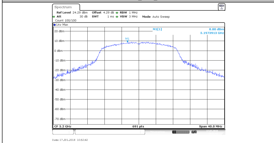
11N20SISO_Ant1_5200
