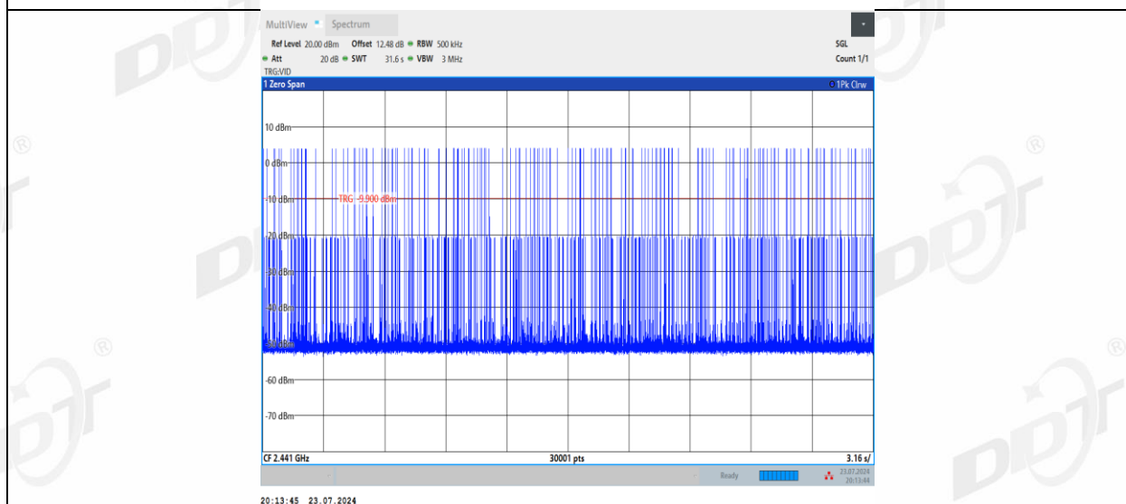
DH3_Ant2_Hop
