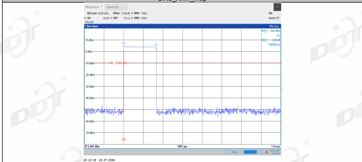
DH3_Ant1_Hop
