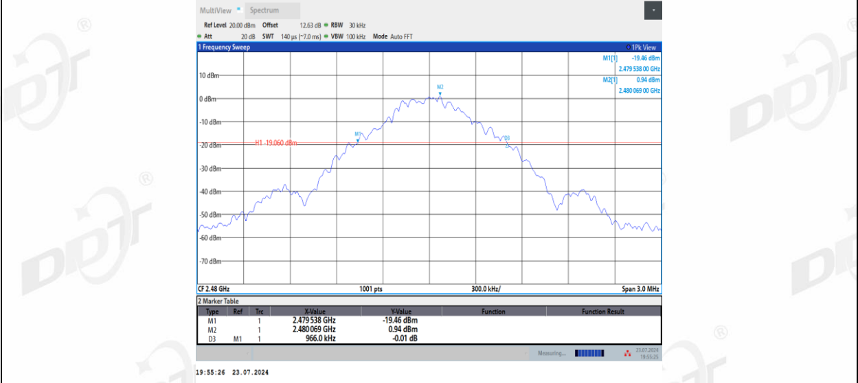
DH5_Ant2_2480
