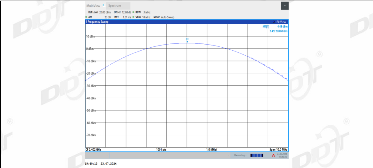
2DH5_Ant2_2402
