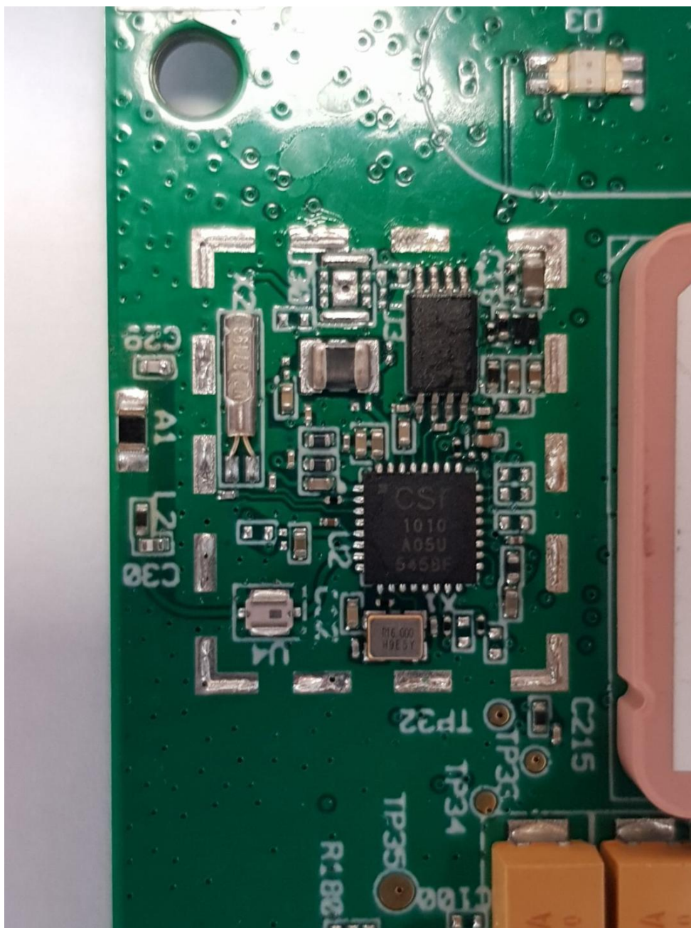
Fig. 11 BLE Circuitry View
