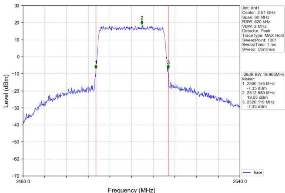
Band7_20MHz_16QAM_LCH_2510MHz_RB_100_0_NTNV
