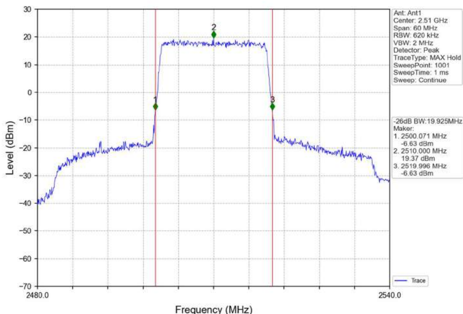
Band7_20MHz_QPSK_LCH_2510MHz_RB_100_0_NTNV
