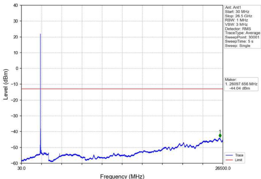
Band7_20MHz_16QAM_MCH_2535MHz_RB_1_0_NTNV
