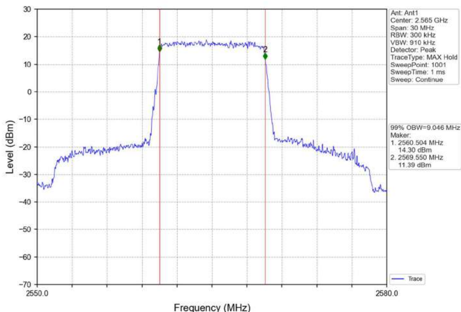
Band7_10MHz_QPSK_HCH_2565MHz_RB_50_0_NTNV
