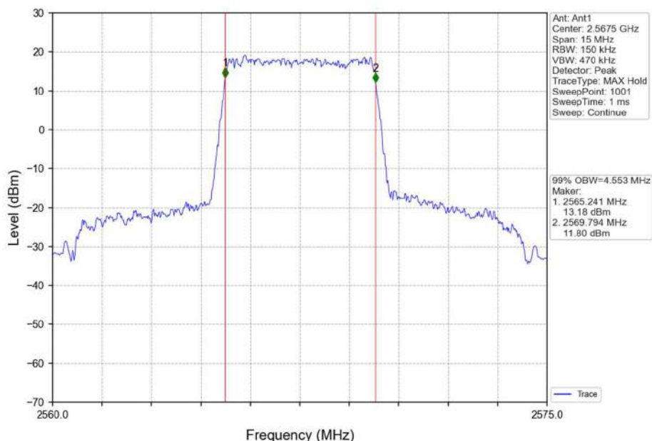
Band7_5MHz_QPSK_HCH_2567.5MHz_RB_25_0_NTNV
