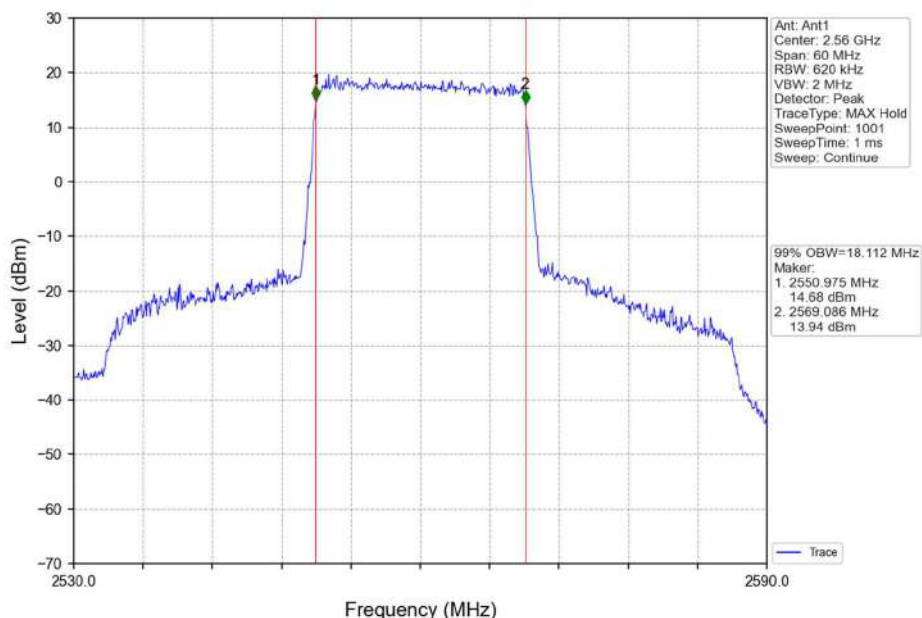
Band7_20MHz_QPSK_HCH_2560MHz_RB_100_0_NTNV
