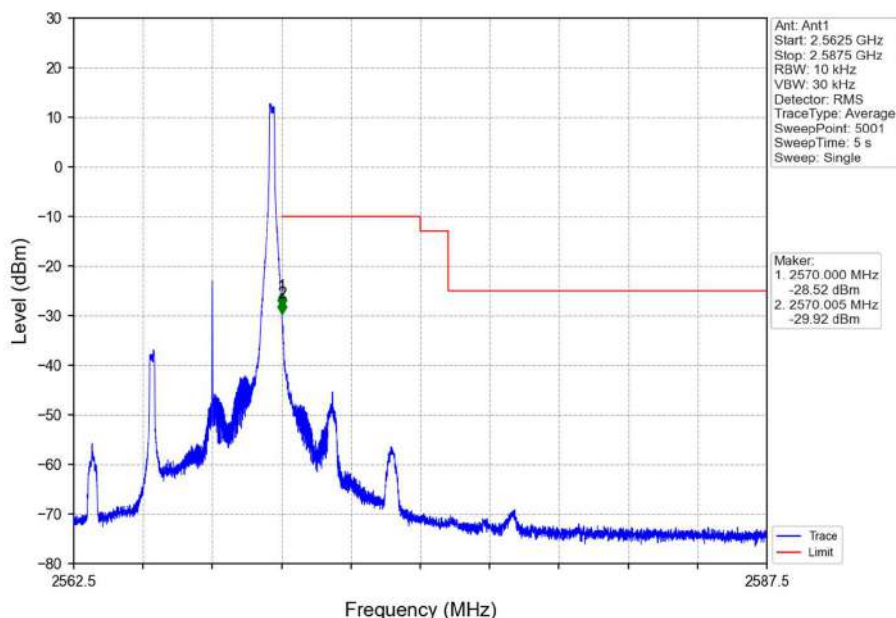
Band7_5MHz_QPSK_HCH_2567.5MHz_RB_1_24_NTNV
