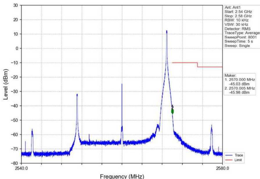
Band7_20MHz_QPSK_HCH_2560MHz_RB_1_99_NTNV
