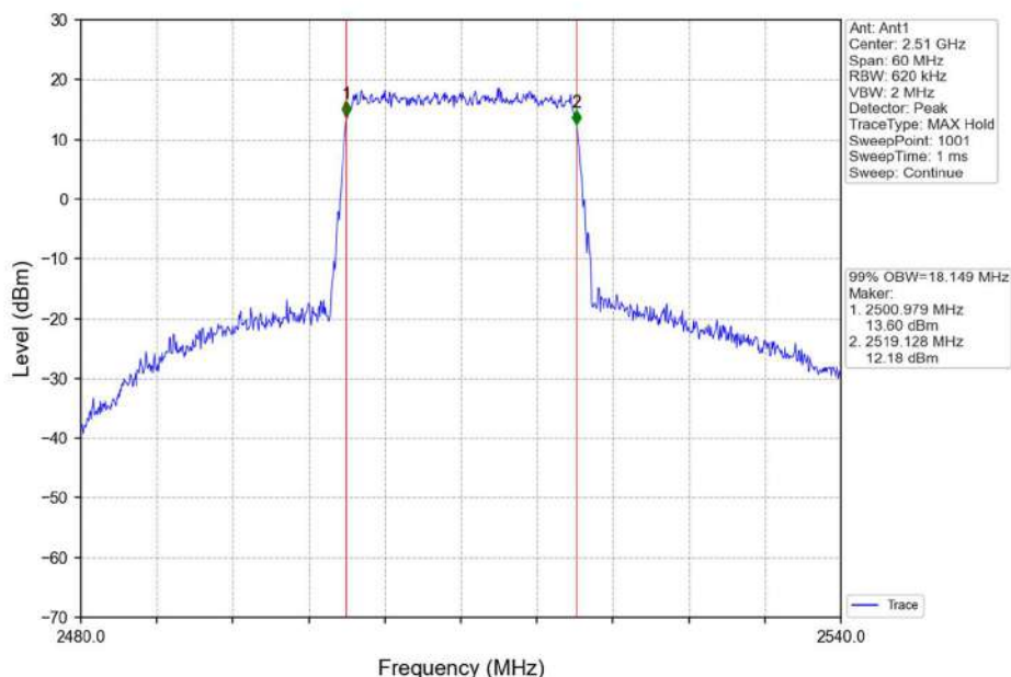
Band7_20MHz_16QAM_LCH_2510MHz_RB_100_0_NTNV
