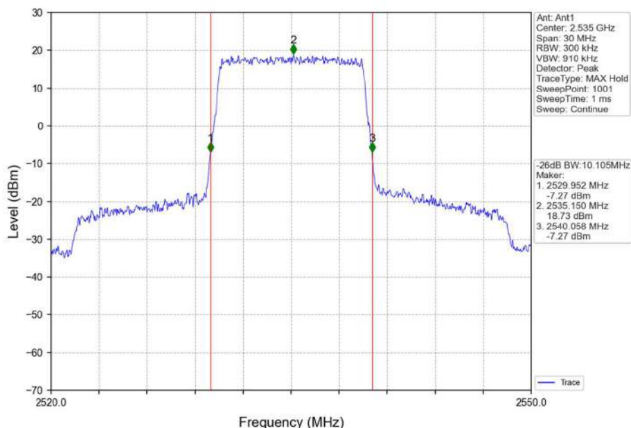
Band7_10MHz_QPSK_MCH_2535MHz_RB_50_0_NTNV
