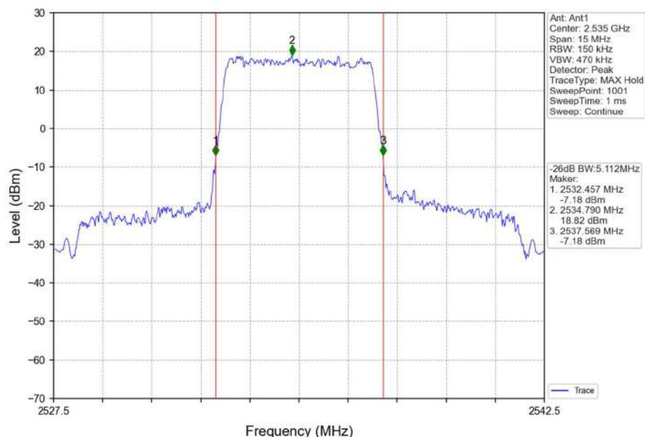
Band7_5MHz_QPSK_MCH_2535MHz_RB_25_0_NTNV
