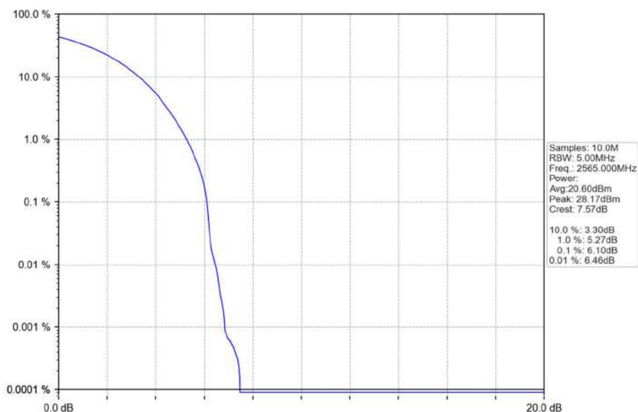
Band7_10MHz_QPSK_HCH_2565MHz_RB_50_0_NTNV
