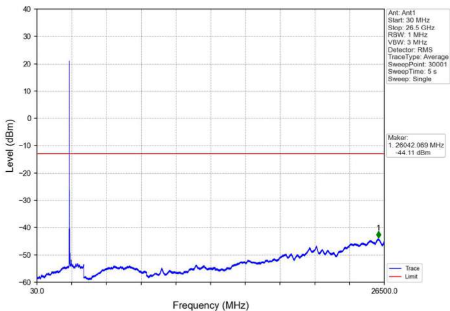
Band7_20MHz_16QAM_LCH_2510MHz_RB_1_0_NTNV
