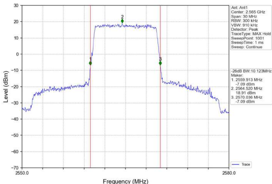
Band7_10MHz_QPSK_HCH_2565MHz_RB_50_0_NTNV
