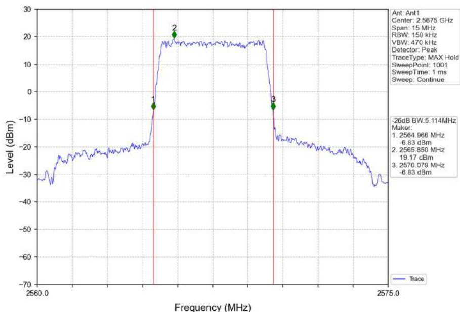
Band7_5MHz_QPSK_HCH_2567.5MHz_RB_25_0_NTNV
