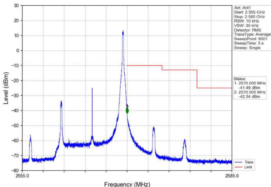
Band7_10MHz_QPSK_HCH_2565MHz_RB_1_49_NTNV
