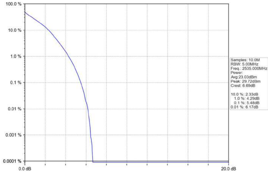
Band7_5MHz_QPSK_MCH_2535MHz_RB_25_0_NTNV
