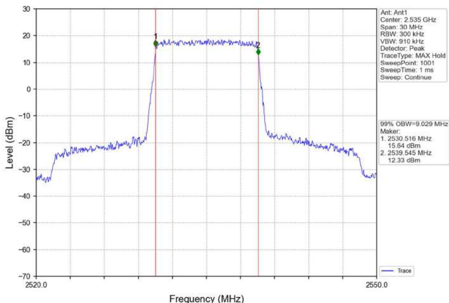
Band7_10MHz_QPSK_MCH_2535MHz_RB_50_0_NTNV
