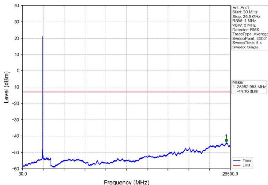
Band7_20MHz_16QAM_HCH_2560MHz_RB_1_0_NTNV
