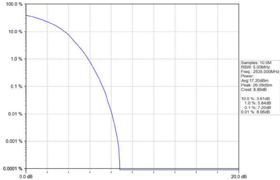
Band7_20MHz_QPSK_MCH_2535MHz_RB_100_0_NTNV
