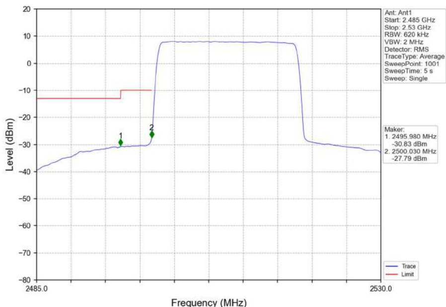
Band7_20MHz_16QAM_LCH_2510MHz_RB_100_0_NTNV
