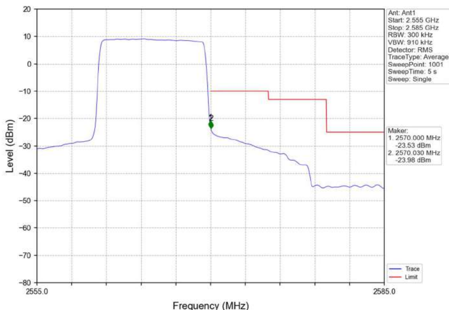
Band7_10MHz_QPSK_HCH_2565MHz_RB_50_0_NTNV
