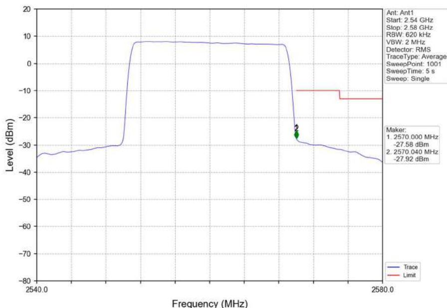
Band7_20MHz_16QAM_HCH_2560MHz_RB_100_0_NTNV
