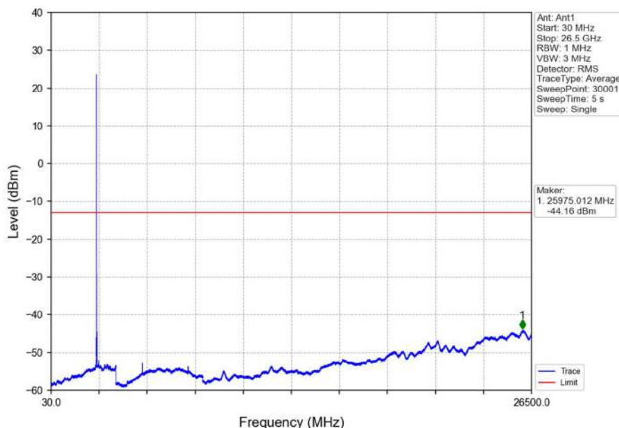
Band7_10MHz_QPSK_MCH_2535MHz_RB_1_0_NTNV
