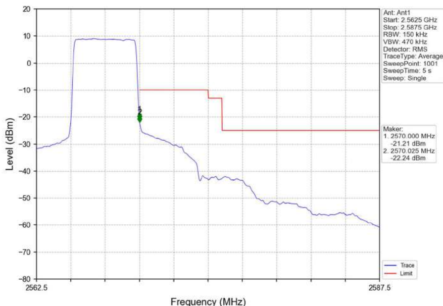
Band7_5MHz_QPSK_HCH_2567.5MHz_RB_25_0_NTNV
