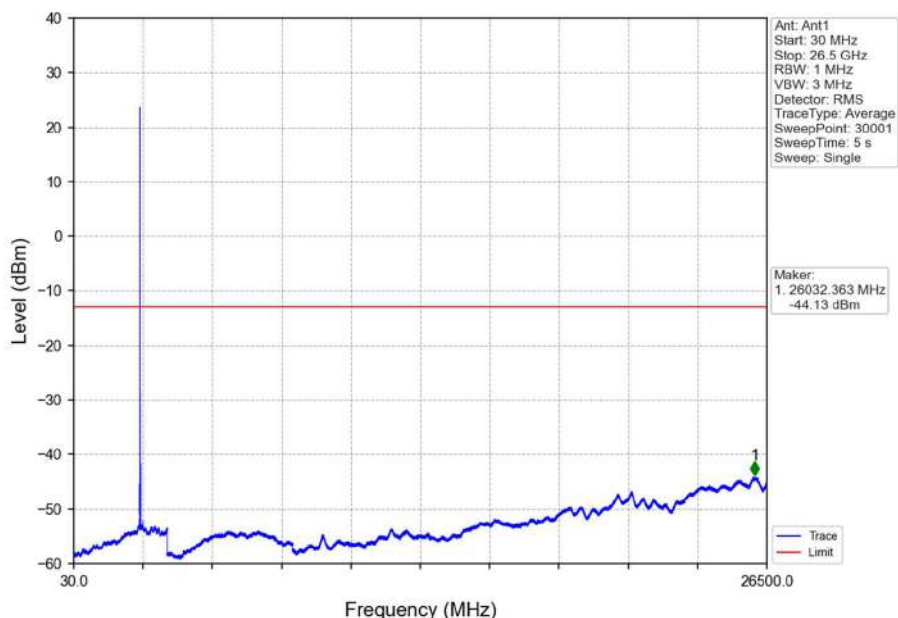
Band7_10MHz_QPSK_HCH_2565MHz_RB_1_0_NTNV
