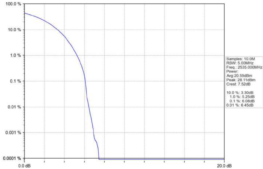
Band7_10MHz_QPSK_MCH_2535MHz_RB_50_0_NTNV
