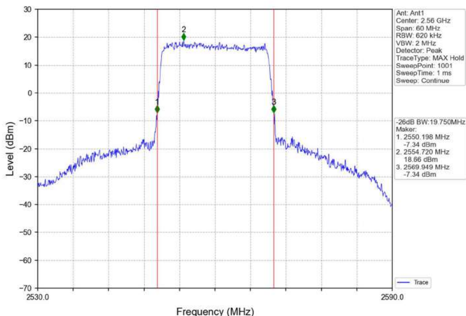
Band7_20MHz_16QAM_HCH_2560MHz_RB_100_0_NTNV
