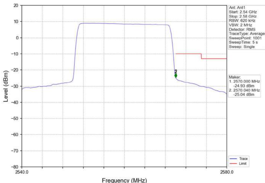
Band7_20MHz_QPSK_HCH_2560MHz_RB_100_0_NTNV
