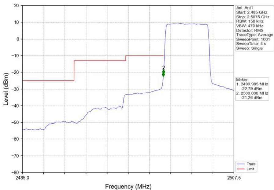
Band7_5MHz_QPSK_LCH_2502.5MHz_RB_25_0_NTNV
