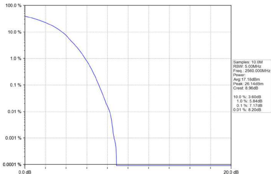
Band7_20MHz_QPSK_HCH_2560MHz_RB_100_0_NTNV
