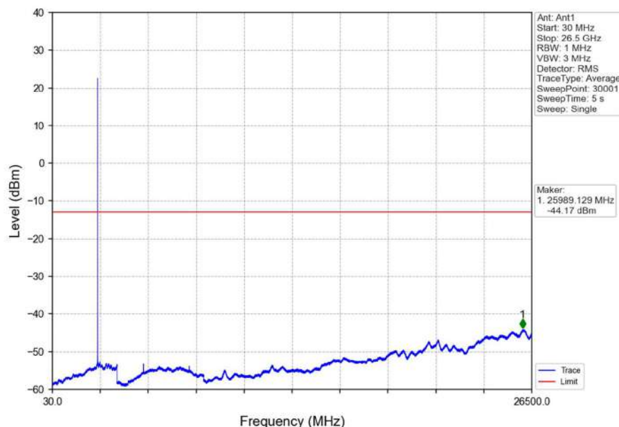
Band7_5MHz_QPSK_MCH_2535MHz_RB_1_0_NTNV
