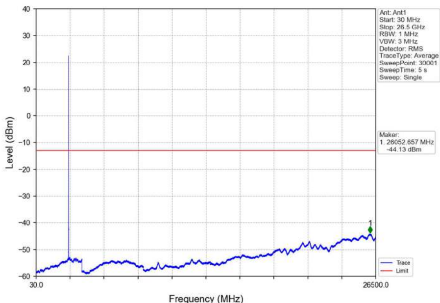
Band7_5MHz_QPSK_HCH_2567.5MHz_RB_1_0_NTNV
