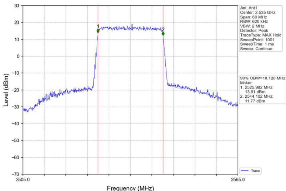
Band7_20MHz_16QAM_MCH_2535MHz_RB_100_0_NTNV
