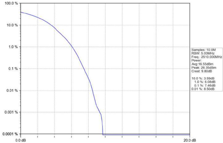
Band7_20MHz_16QAM_LCH_2510MHz_RB_100_0_NTNV
