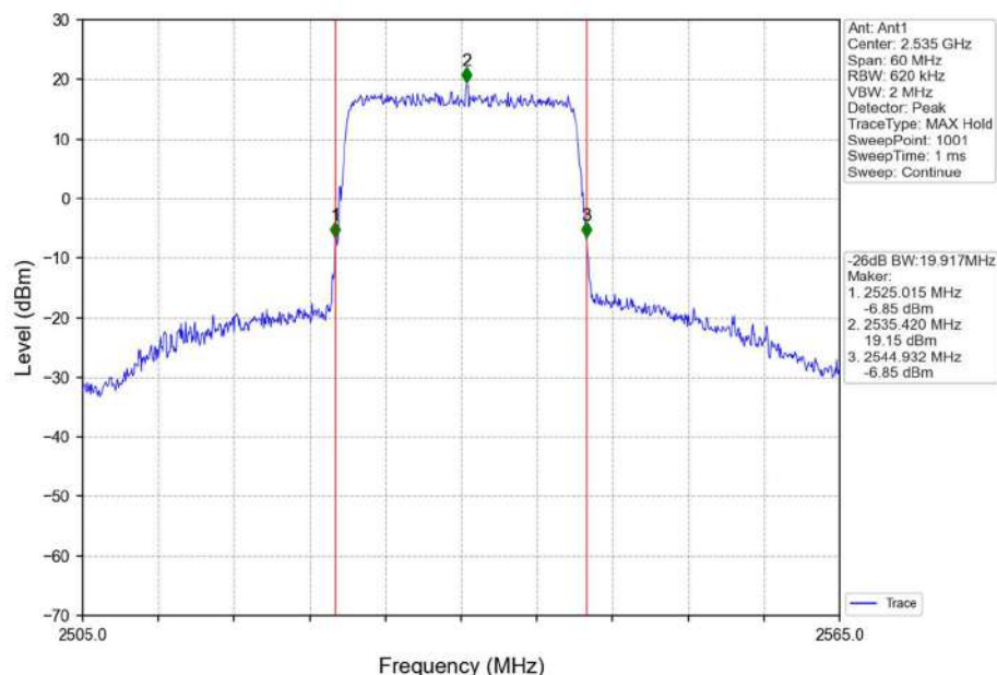
Band7_20MHz_16QAM_MCH_2535MHz_RB_100_0_NTNV
