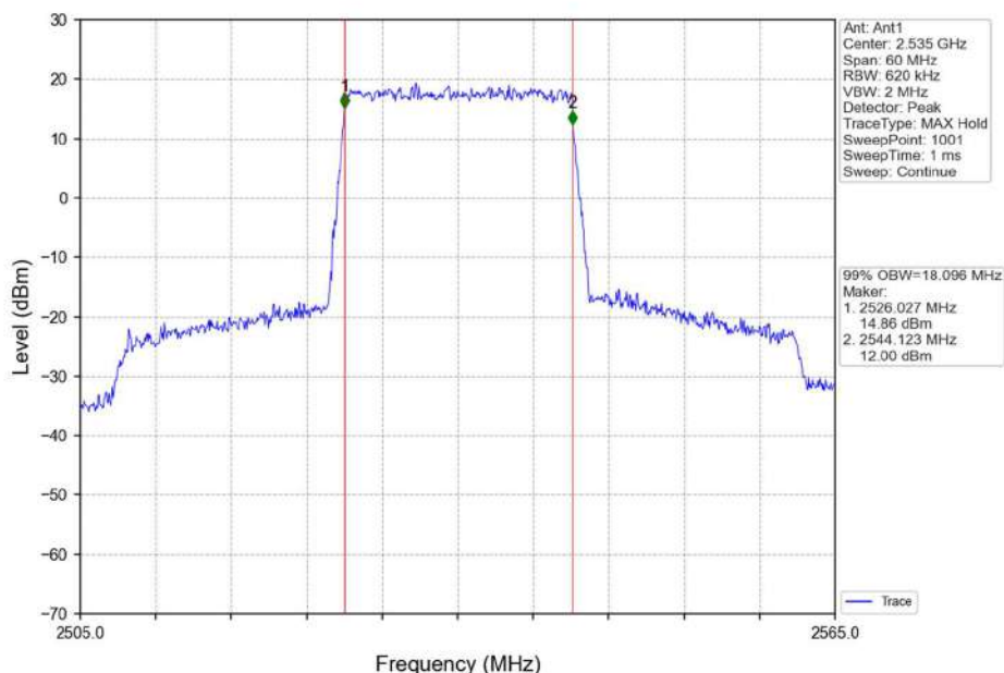
Band7_20MHz_QPSK_MCH_2535MHz_RB_100_0_NTNV
