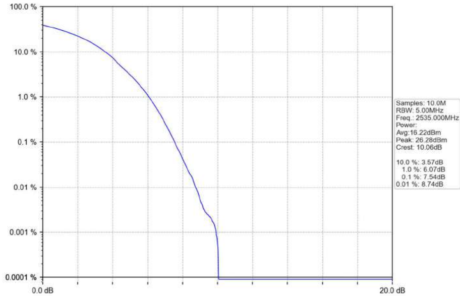
Band7_20MHz_16QAM_MCH_2535MHz_RB_100_0_NTNV
