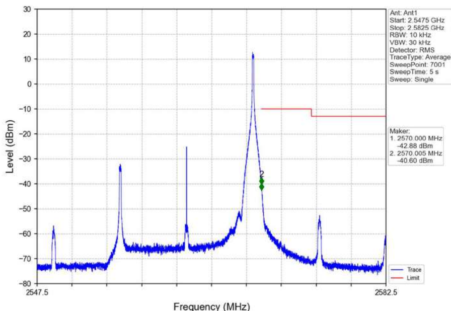
Band7_15MHz_QPSK_HCH_2562.5MHz_RB_1_74_NTNV
