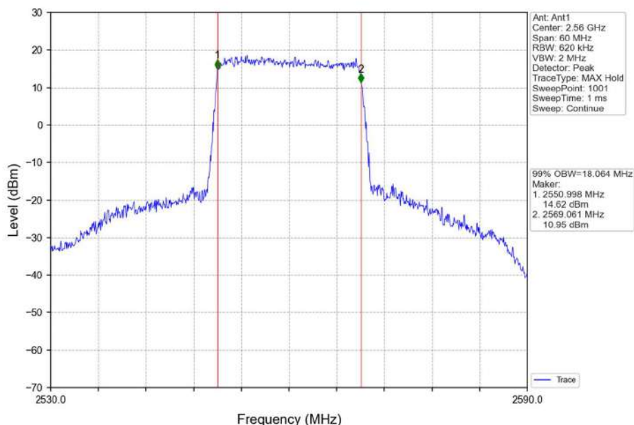
Band7_20MHz_16QAM_HCH_2560MHz_RB_100_0_NTNV
