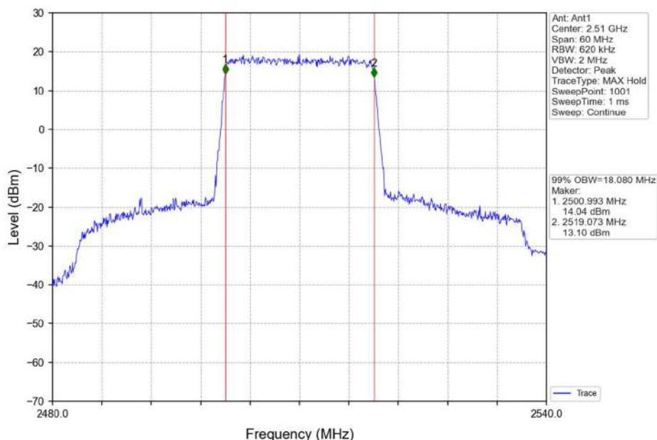
Band7_20MHz_QPSK_LCH_2510MHz_RB_100_0_NTNV
