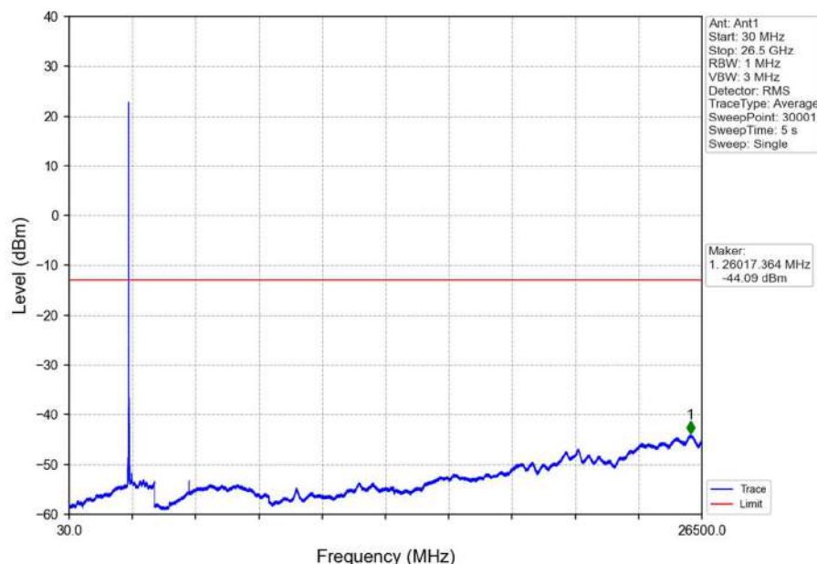
Band7_20MHz_QPSK_MCH_2535MHz_RB_1_0_NTNV
