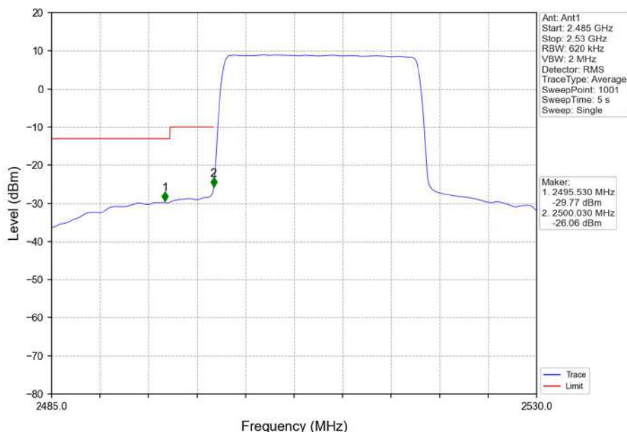
Band7_20MHz_QPSK_LCH_2510MHz_RB_100_0_NTNV
