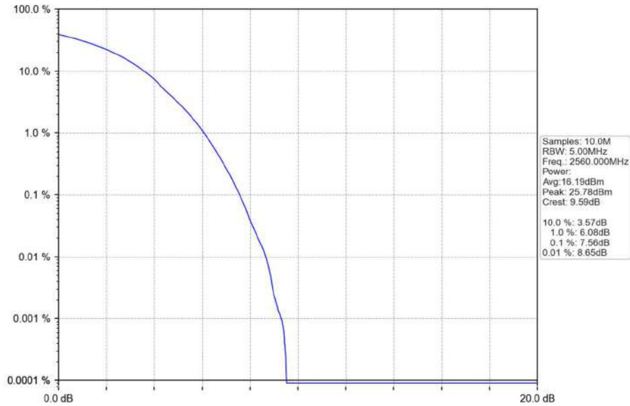
Band7_20MHz_16QAM_HCH_2560MHz_RB_100_0_NTNV
