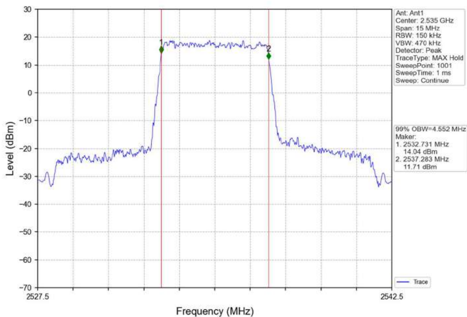
Band7_5MHz_QPSK_MCH_2535MHz_RB_25_0_NTNV
