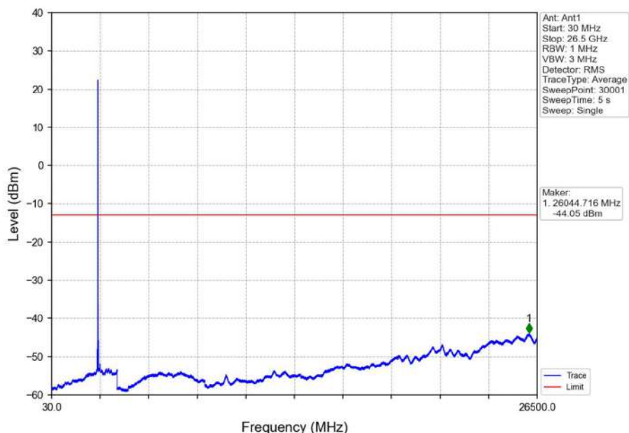
Band7_20MHz_QPSK_HCH_2560MHz_RB_1_0_NTNV
