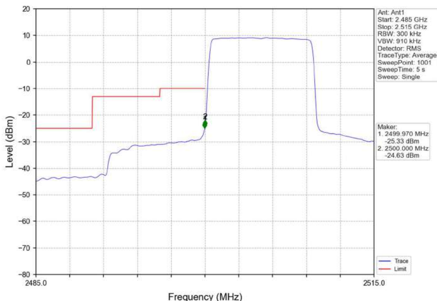
Band7_10MHz_QPSK_LCH_2505MHz_RB_50_0_NTNV
