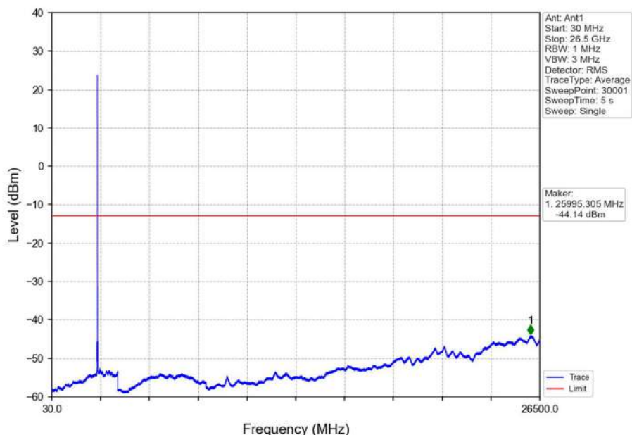
Band7_10MHz_QPSK_LCH_2505MHz_RB_1_0_NTNV
