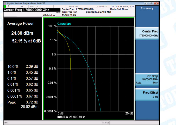
Band4-10MHz-QPSK-20350-1RB#0-PASS
