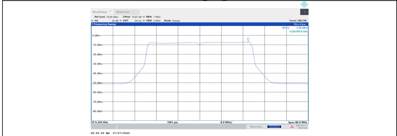
11BE40MIMO_Ant1_6245
