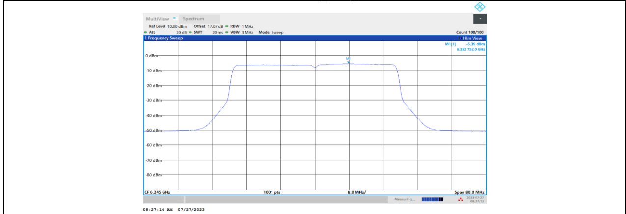
11BE40MIMO_Ant4_6245
