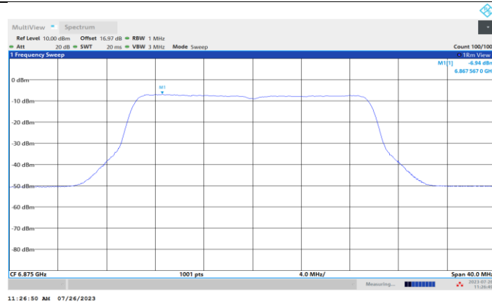
11BE20MIMO_Ant2_6875
