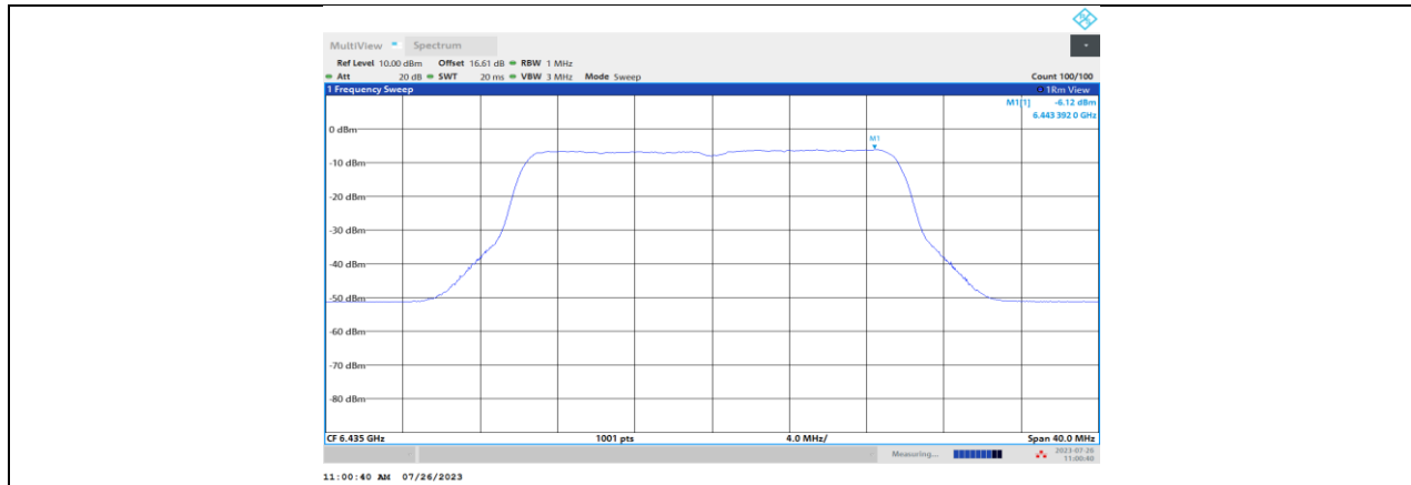
11BE20MIMO_Ant4_6435
