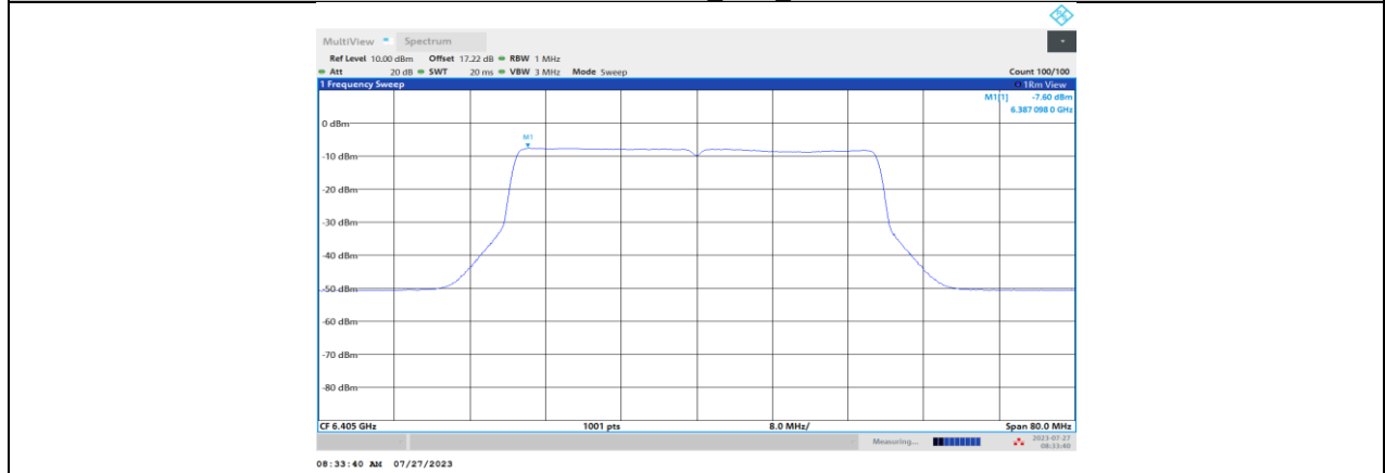
11BE40MIMO_Ant1_6405
