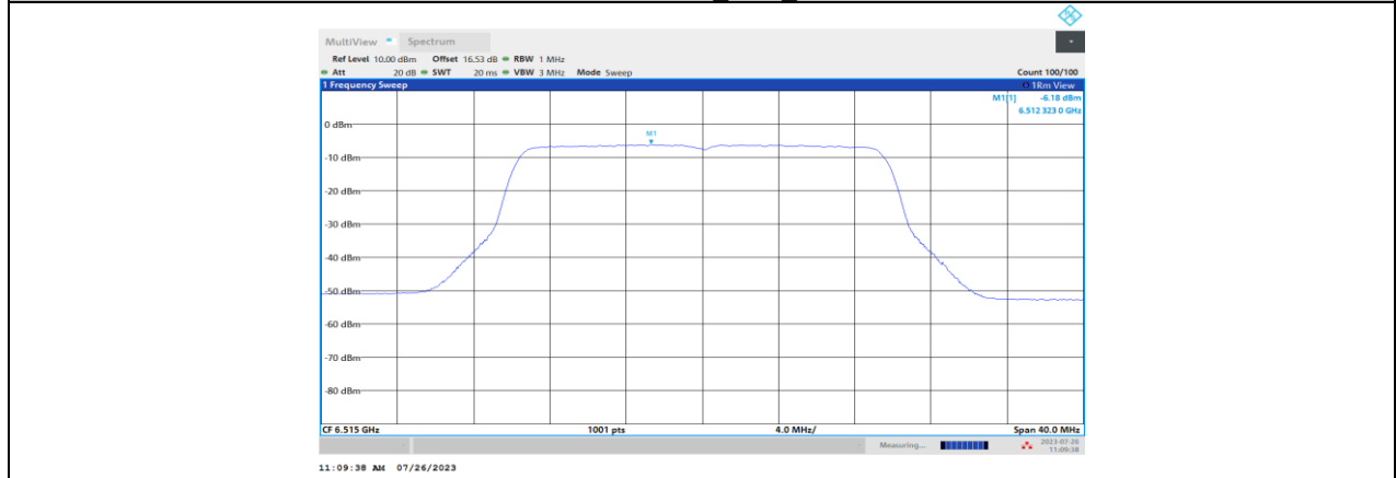
11BE20MIMO_Ant3_6515
