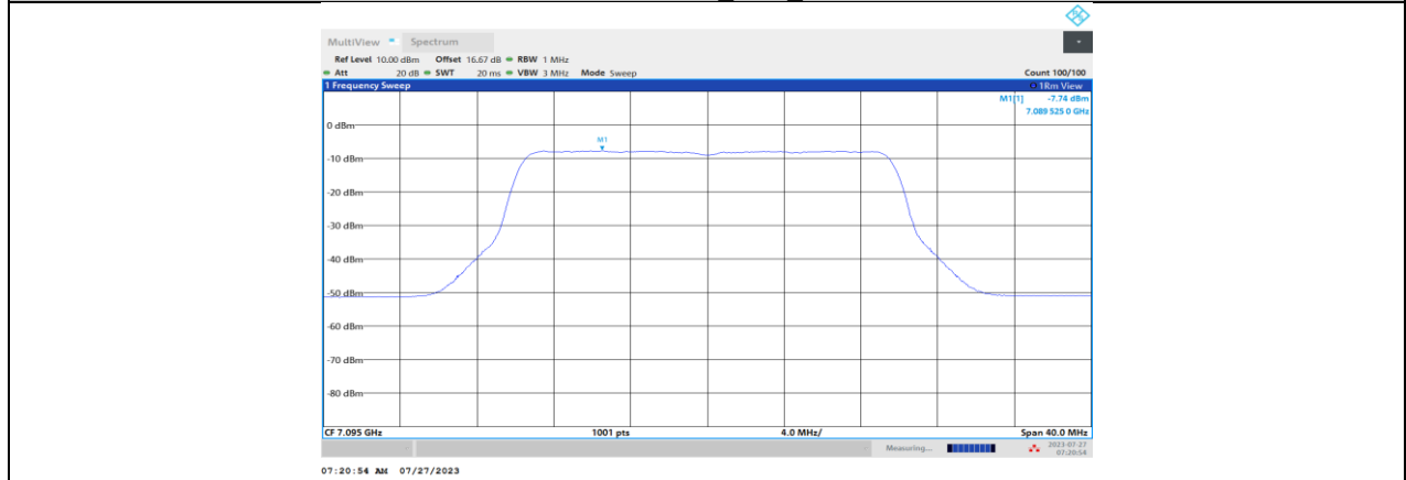
11BE20MIMO_Ant1_7095
