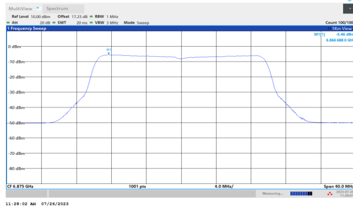
11BE20MIMO_Ant4_6875
