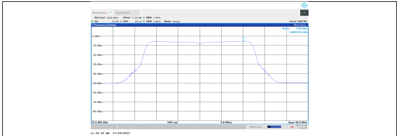
11BE20MIMO_Ant4_6895
