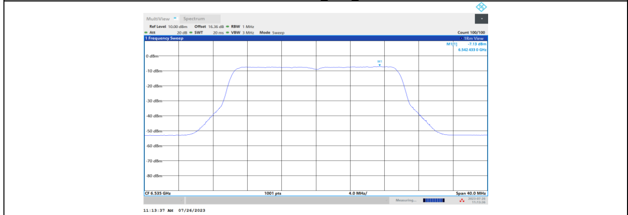
11BE20MIMO_Ant2_6535
