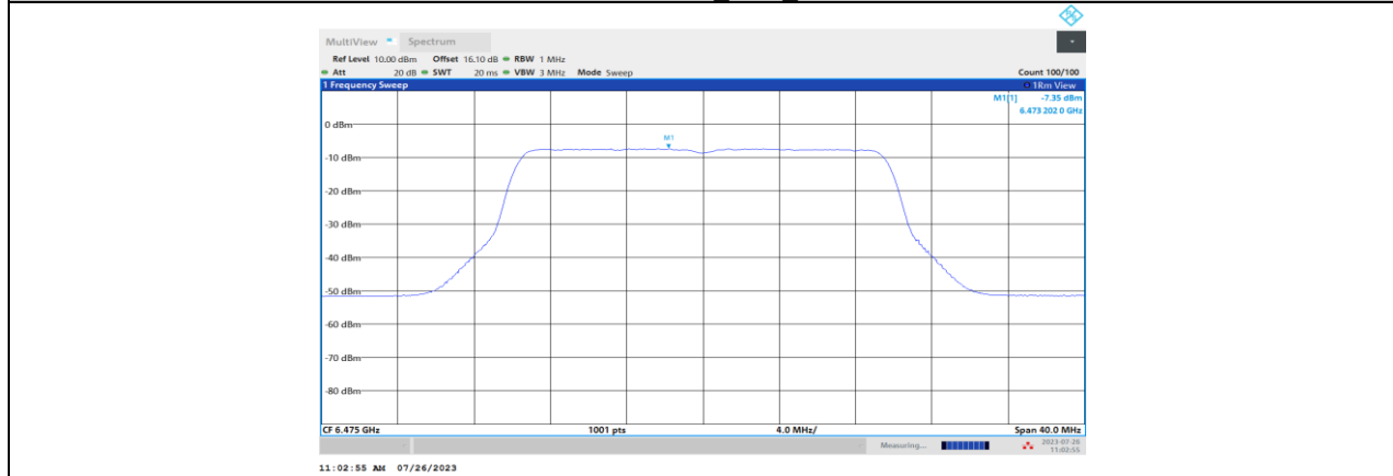
11BE20MIMO_Ant1_6475
