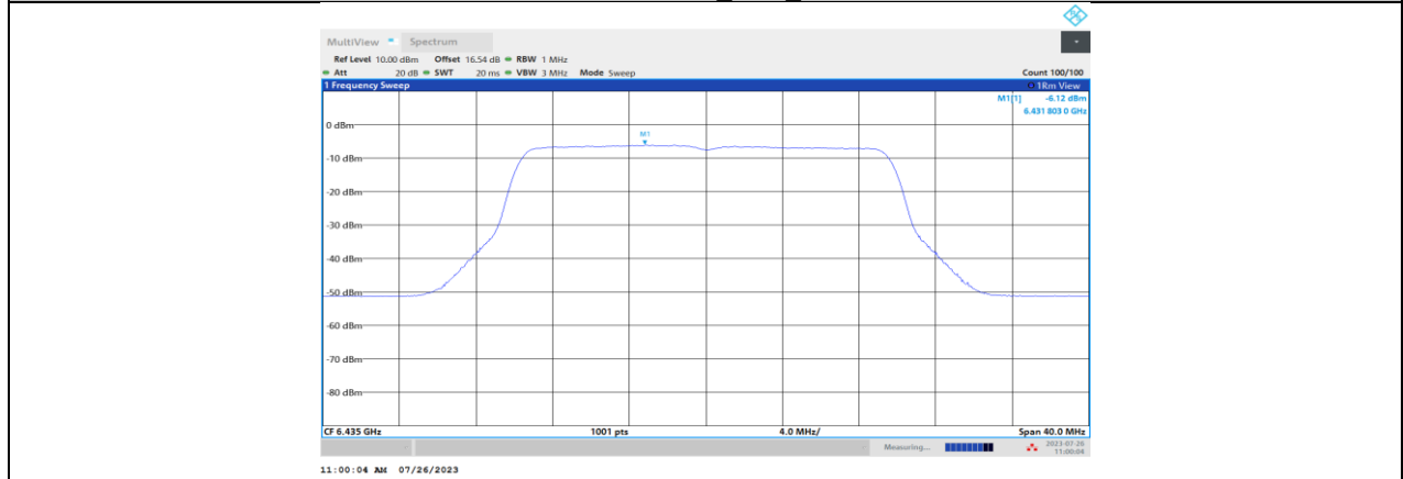
11BE20MIMO_Ant3_6435
