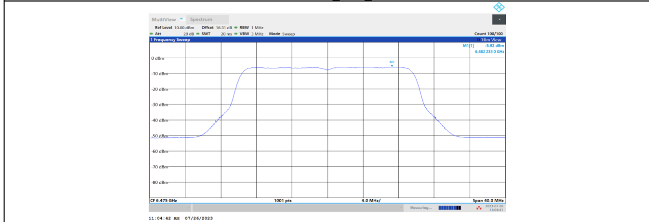
11BE20MIMO_Ant4_6475
