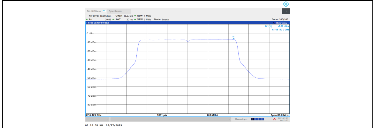
11BE40MIMO_Ant2_6125
