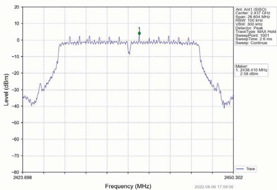
802.11n(HT20)_MCH_2437MHz_Ant1 (SISO)_NTNV
