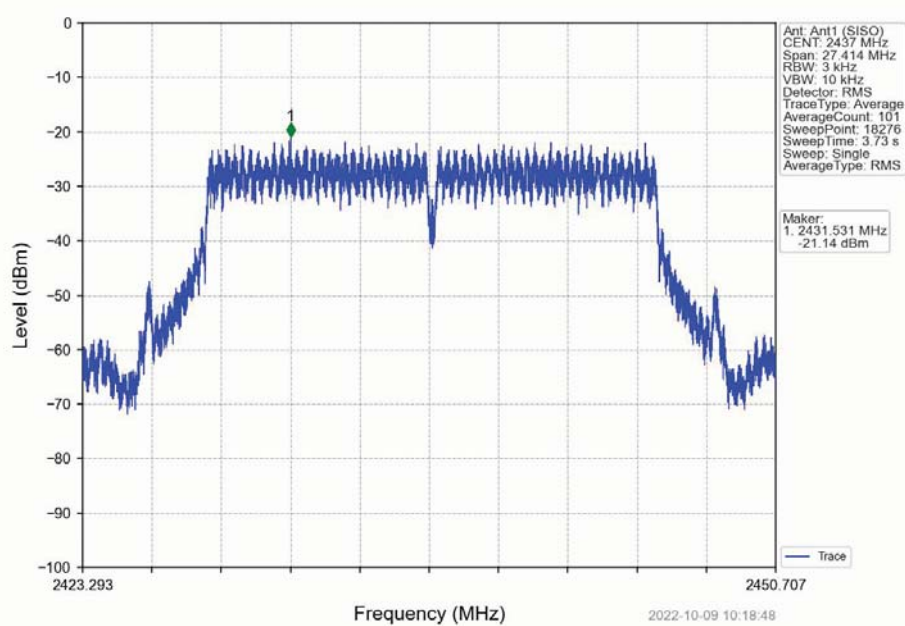
802.11n(HT20)_MCH_2437MHz_Ant1 (SISO)_NTNV
