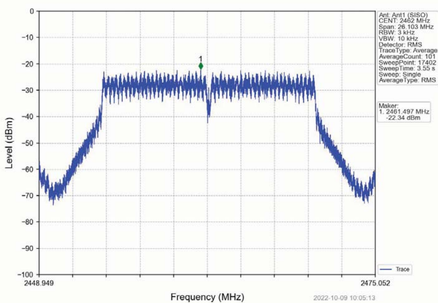
802.11g_HCH_2462MHz_Ant1 (SISO)_NTNV
