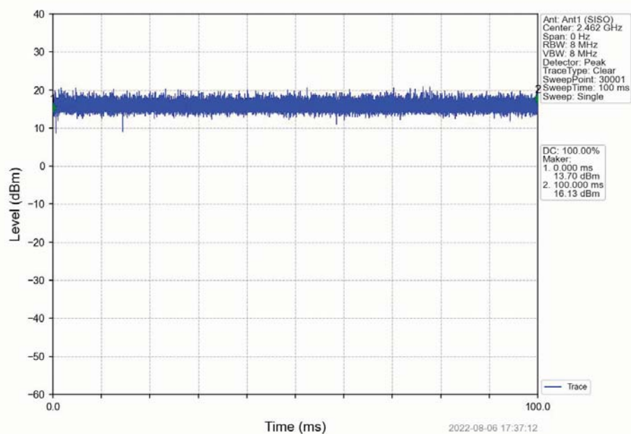
802.11g_HCH_2462MHz_Ant1 (SISO)_NTNV
