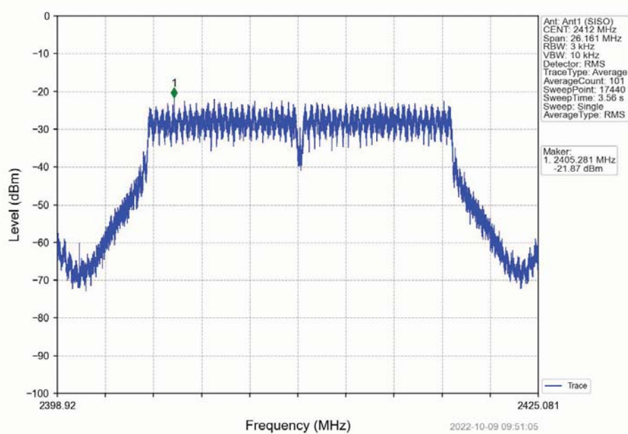
802.11g_LCH_2412MHz_Ant1 (SISO)_NTNV
