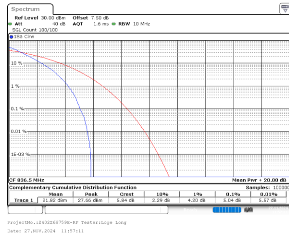
10MHz_Middle_16QAM_50@0
