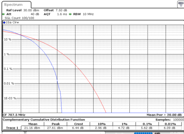
10MHz_Middle_16QAM_50@0
