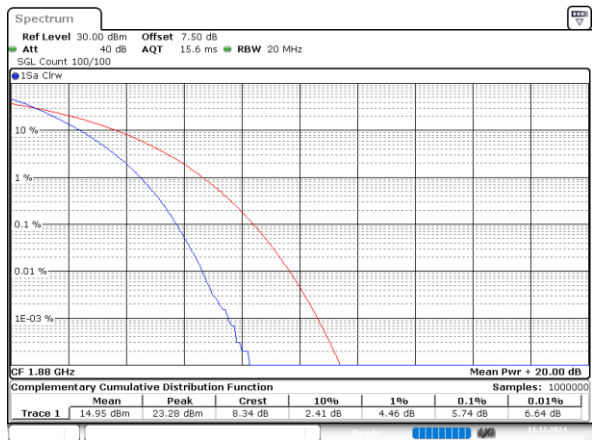
20MHz_Middle_QPSK_100@0
