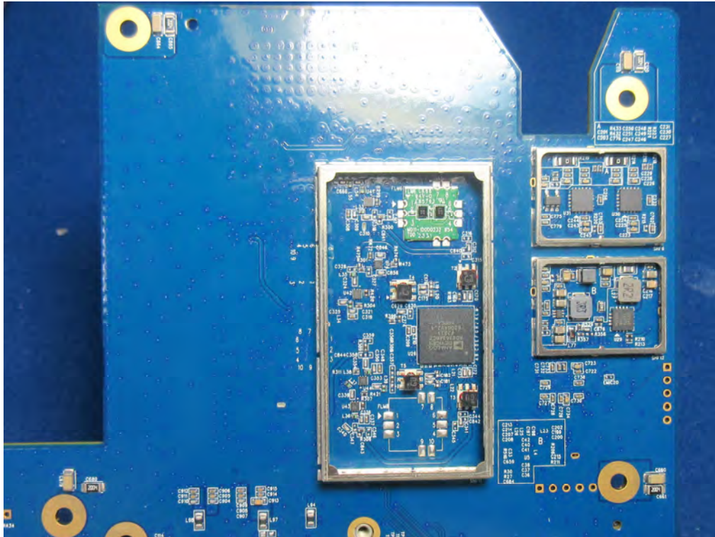
(52) EUT Photo
