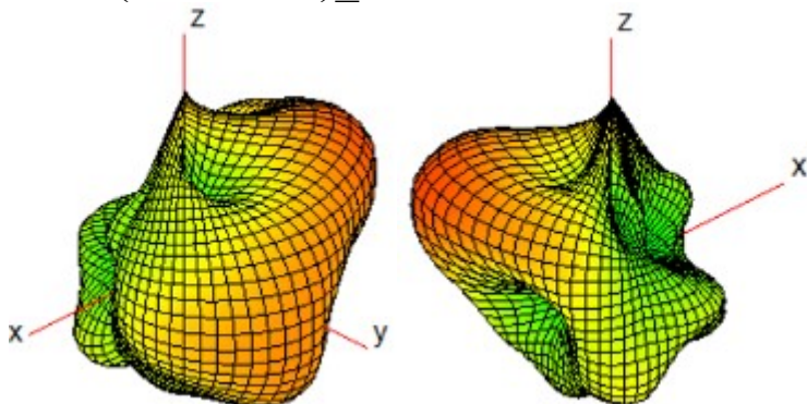
Ant 8(WiFi1/BT)_6200MHz
