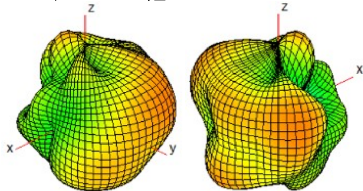
Ant 8(WiFi1/BT)_7000MHz
