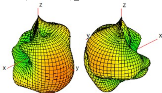
Ant 8(WiFi1/BT)_6200MHz
