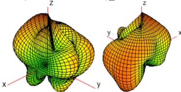
Ant 8(WiFi1/BT)_2450MHz
