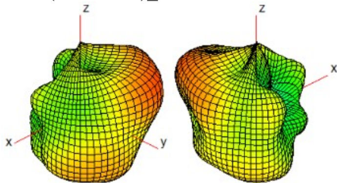
Ant 8(WiFi1/BT)_7000MHz
