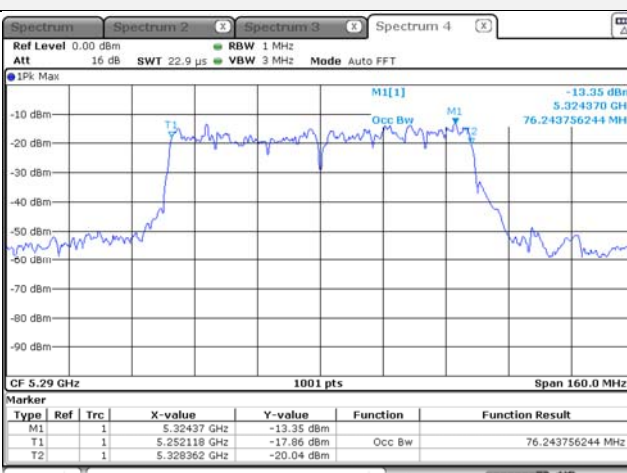
802.11ac(VHT80) - 5 290 MHz
