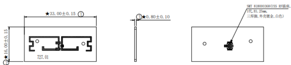
反面(SMTIPEX+黑色油墨)
