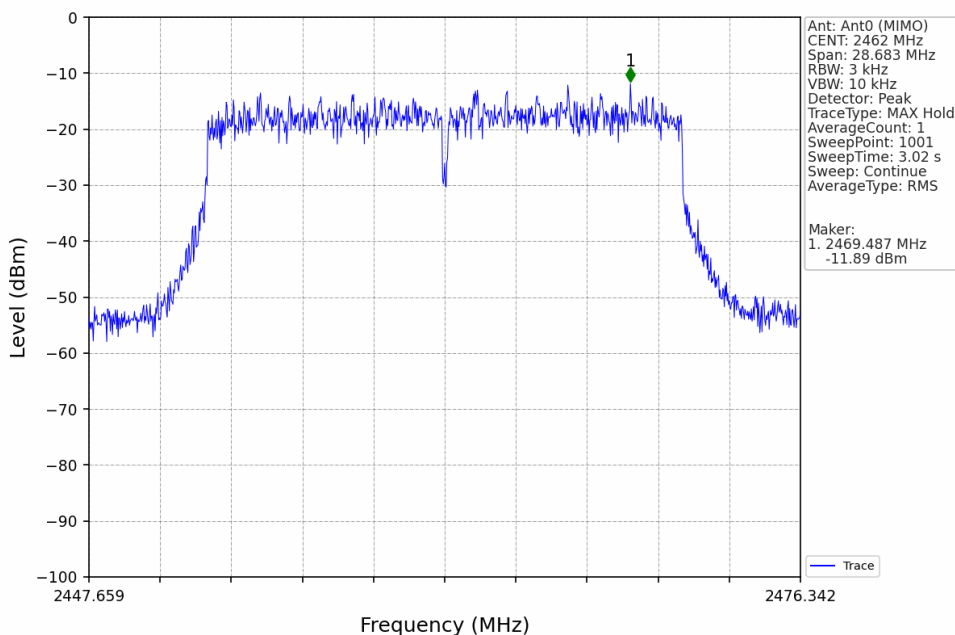
802.11ax(HEW20)_HCH_2462MHz_RU242_Left_Ant0 (MIMO)_NTNV
