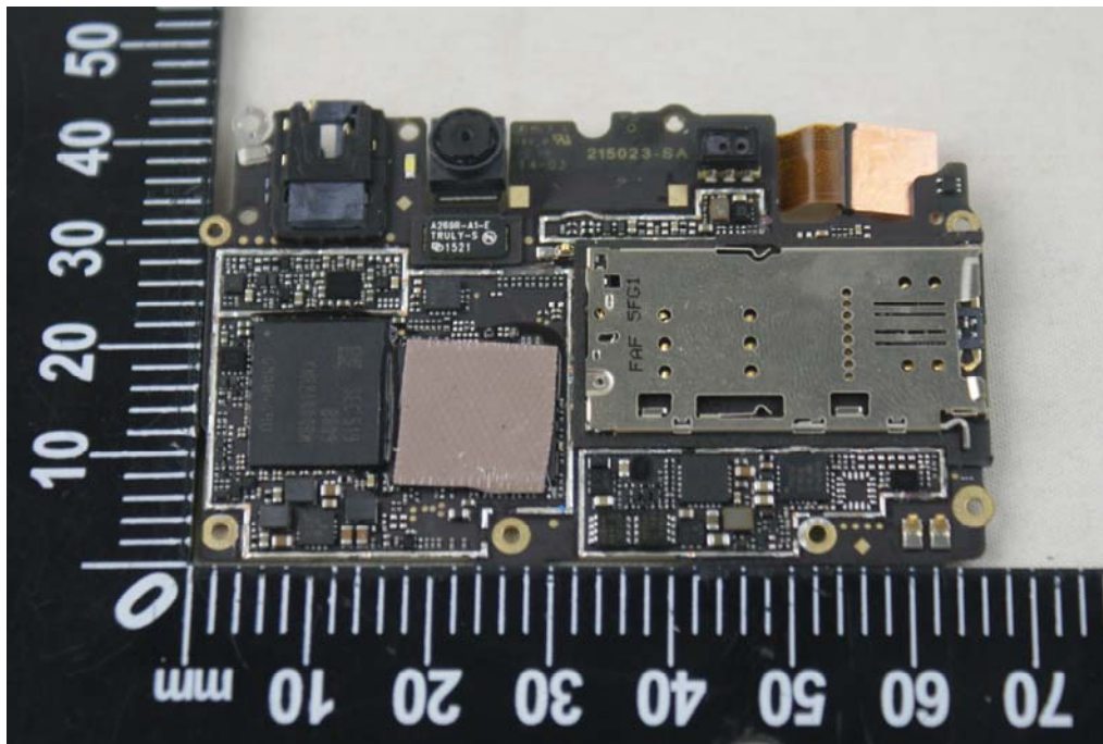
EUT Photo 9
