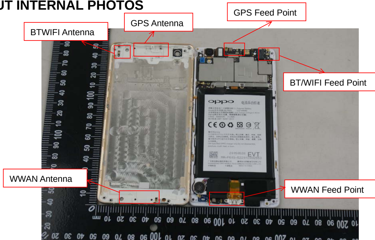
EUT Photo 1
