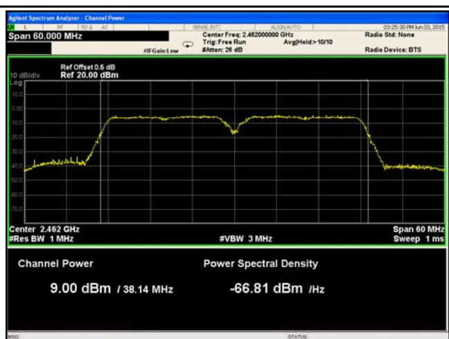
802.11n40 - AV Output power - High CH 2462
