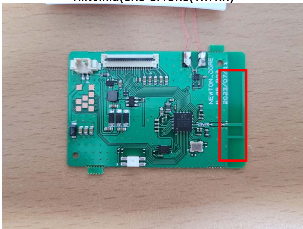
Antenna(SRD 2.4GHz(TX/RX))
