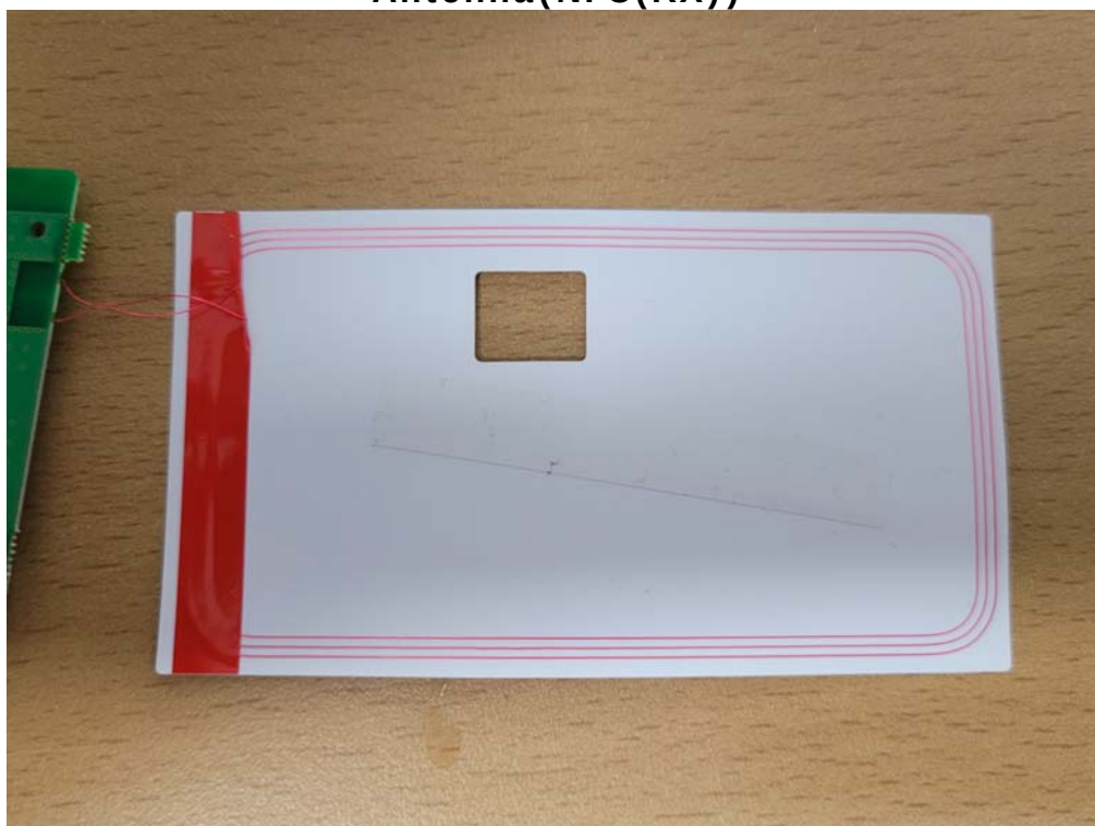
Antenna(NFC(RX))
