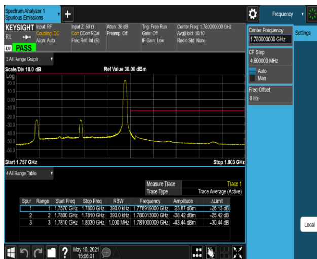
Band66-20MHz-QPSK-132572-1RB#99
