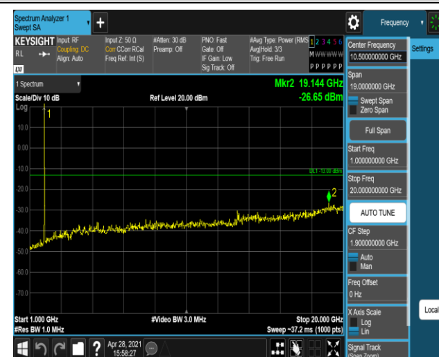
Band2-20MHz-16QAM-19100-1RB#0-Range2:1000~20
