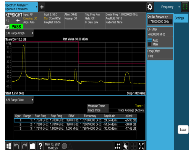
Band66-20MHz-QPSK-132572-100RB#0
