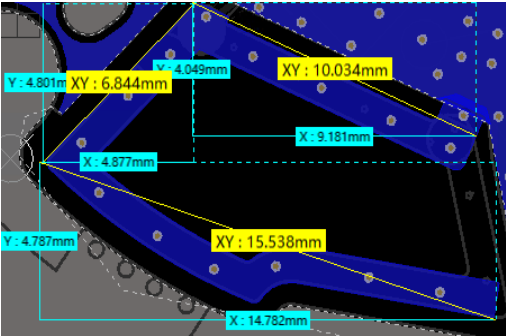
天线尺寸/ANT Size
