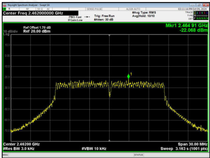
802.11g - CH11
