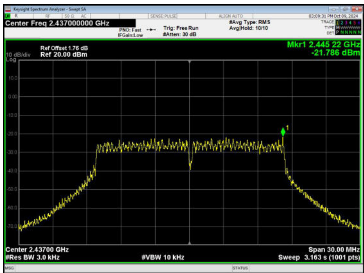
802.11g - CH06
