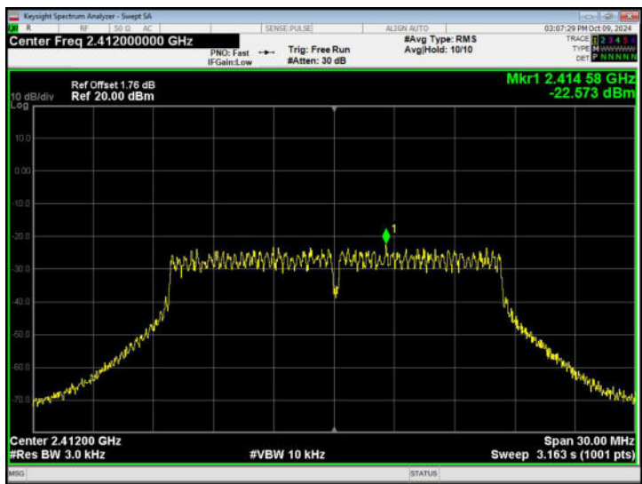
802.11g - CH01
