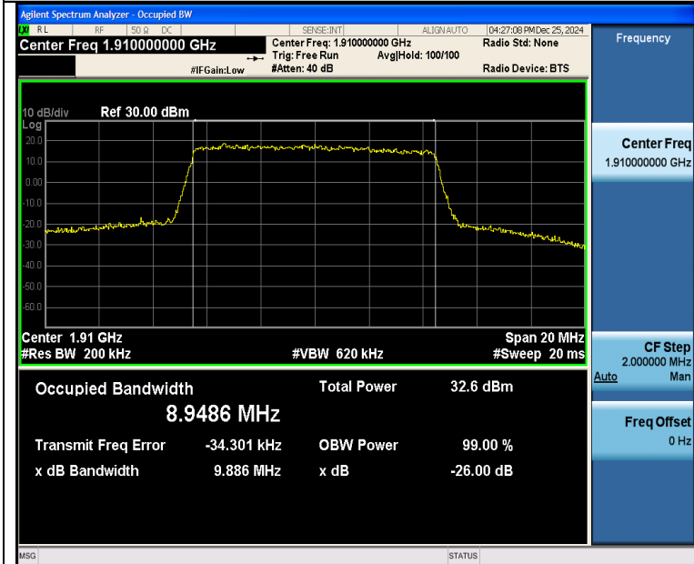
Band25-10MHz-QPSK-26640-50RB#0-PASS
