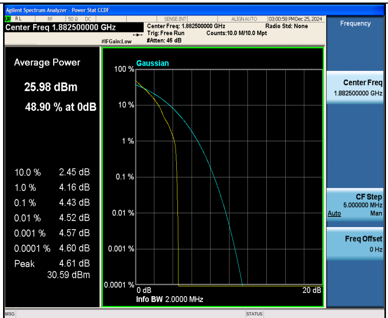
Band25-1.4MHz-QPSK-26365-1RB#0-PASS
