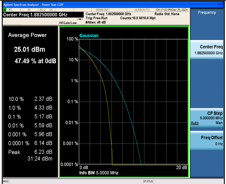
Band25-5MHz-QPSK-26365-25RB#0-PASS
