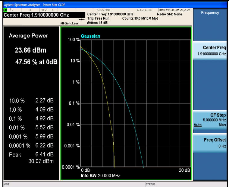
Band25-10MHz-QPSK-26640-50RB#0-PASS
