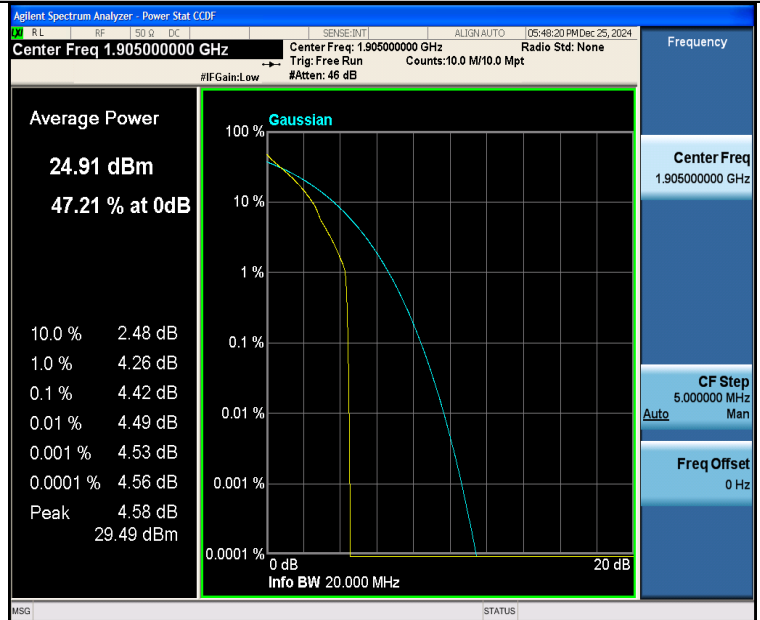
Band25-20MHz-QPSK-26590-1RB#0-PASS
