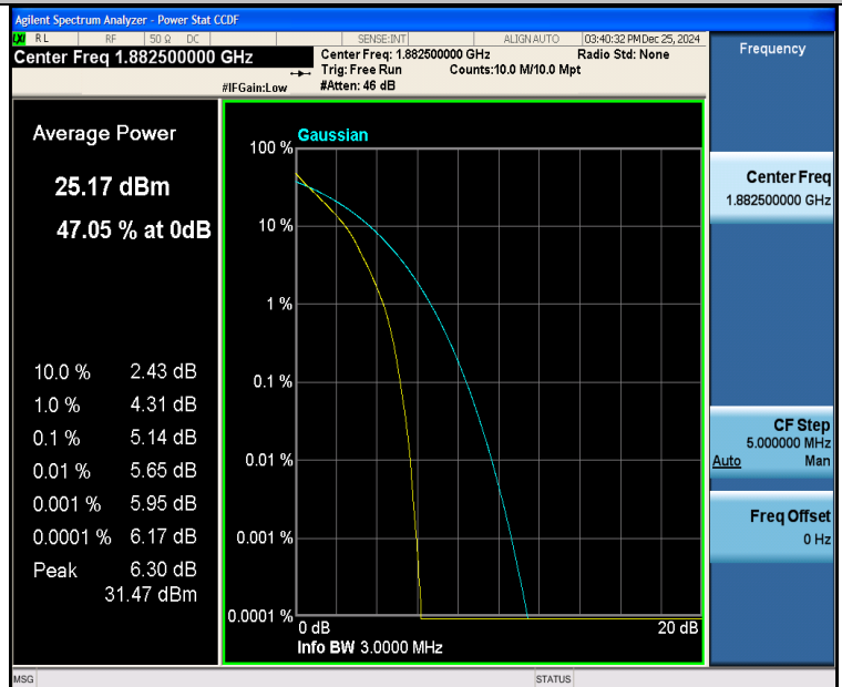
Band25-3MHz-QPSK-26365-15RB#0-PASS
