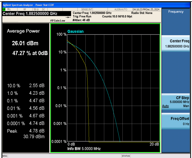
Band25-5MHz-QPSK-26365-1RB#0-PASS
