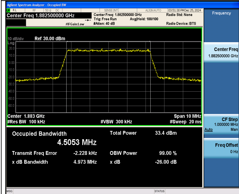
Band25-5MHz-QPSK-26365-25RB#0-PASS
