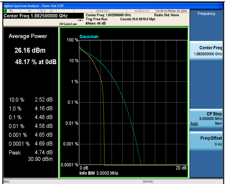
Band25-3MHz-QPSK-26365-1RB#0-PASS
