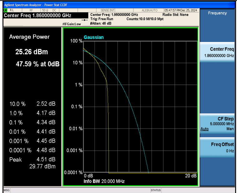
Band25-20MHz-QPSK-26140-1RB#0-PASS
