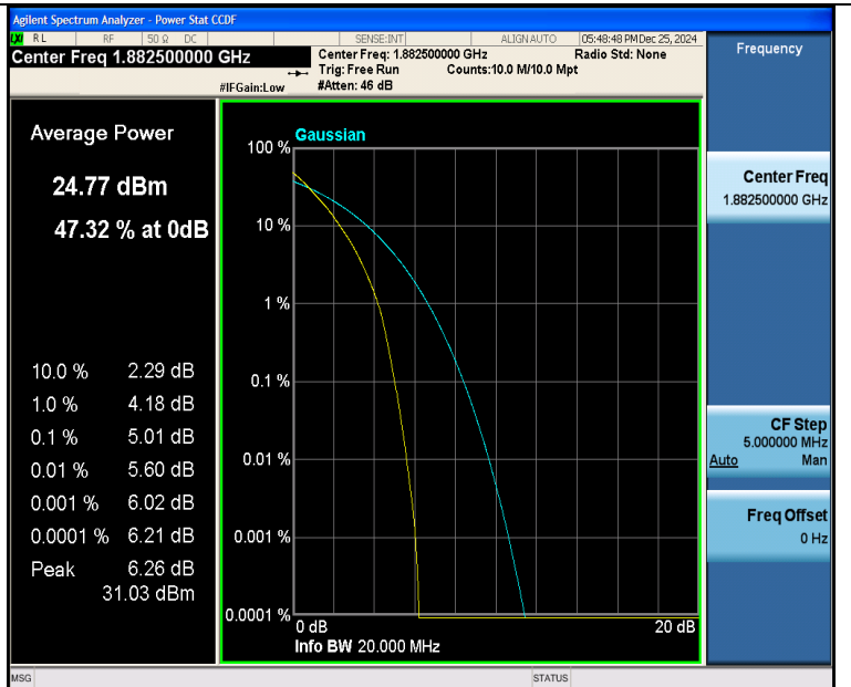
Band25-20MHz-QPSK-26365-100RB#0-PASS
