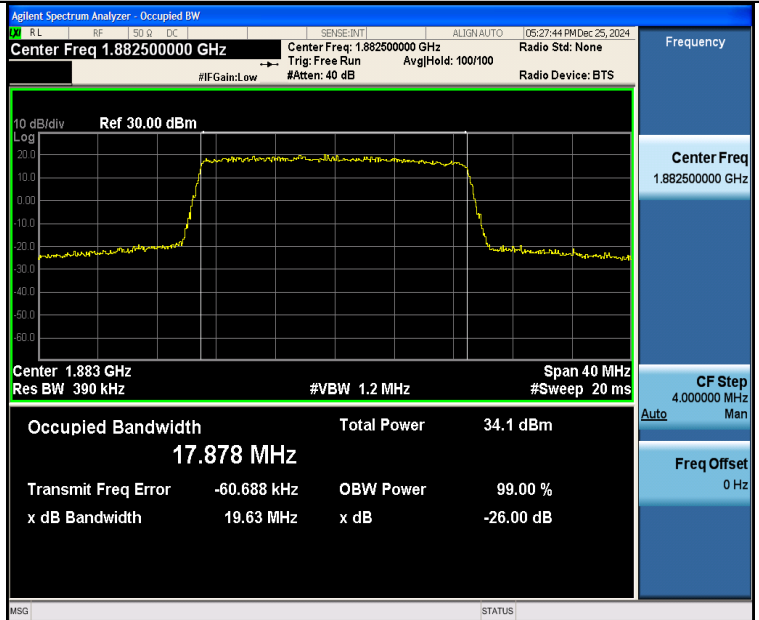
Band25-20MHz-QPSK-26365-100RB#0-PASS
