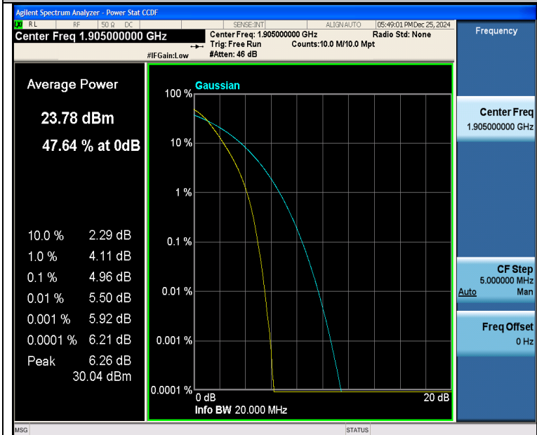
Band25-20MHz-QPSK-26590-100RB#0-PASS
