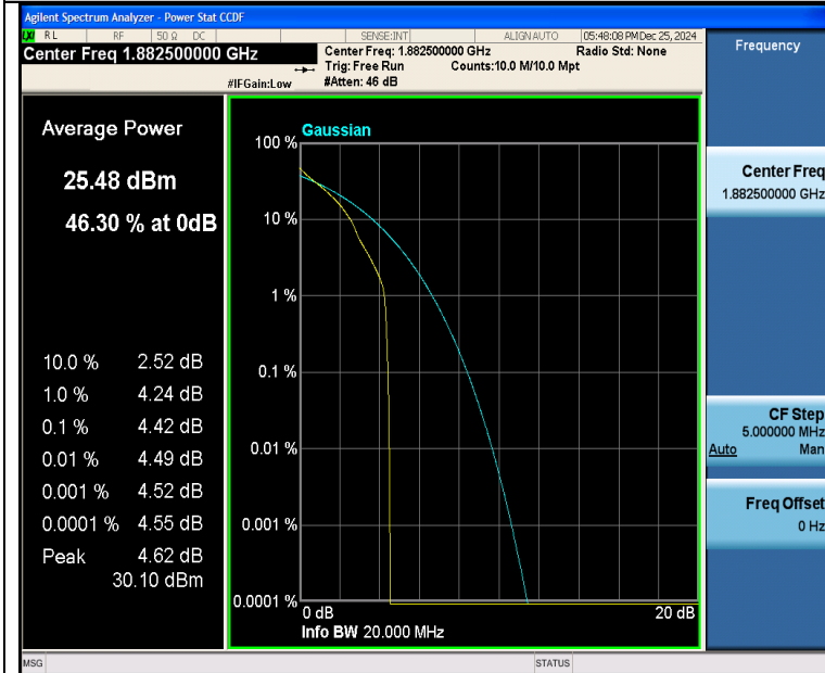
Band25-20MHz-QPSK-26365-1RB#0-PASS
