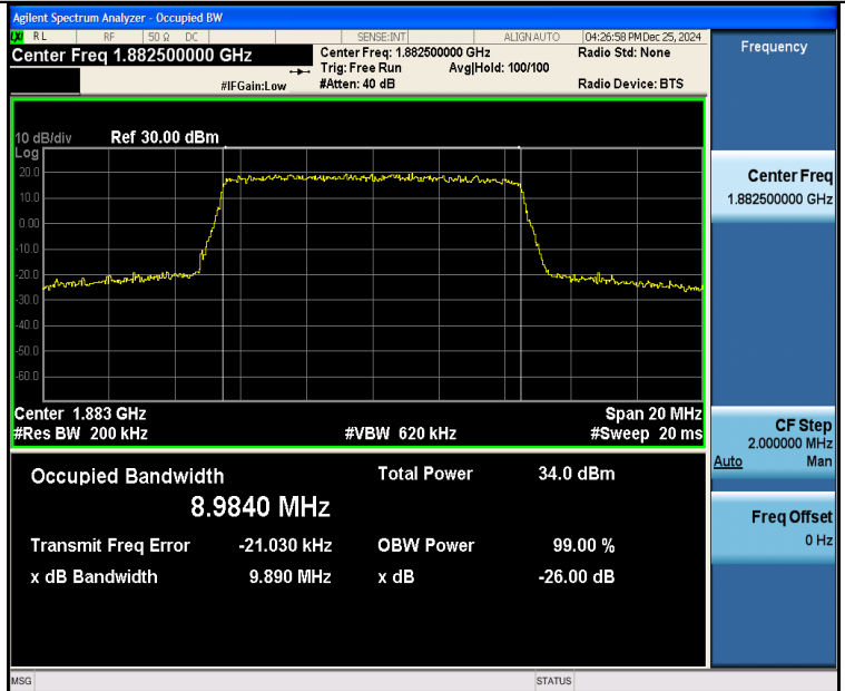
Band25-10MHz-QPSK-26365-50RB#0-PASS
