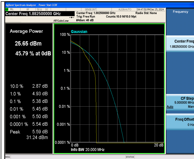
Band25-10MHz-16QAM-26365-1RB#0-PASS
