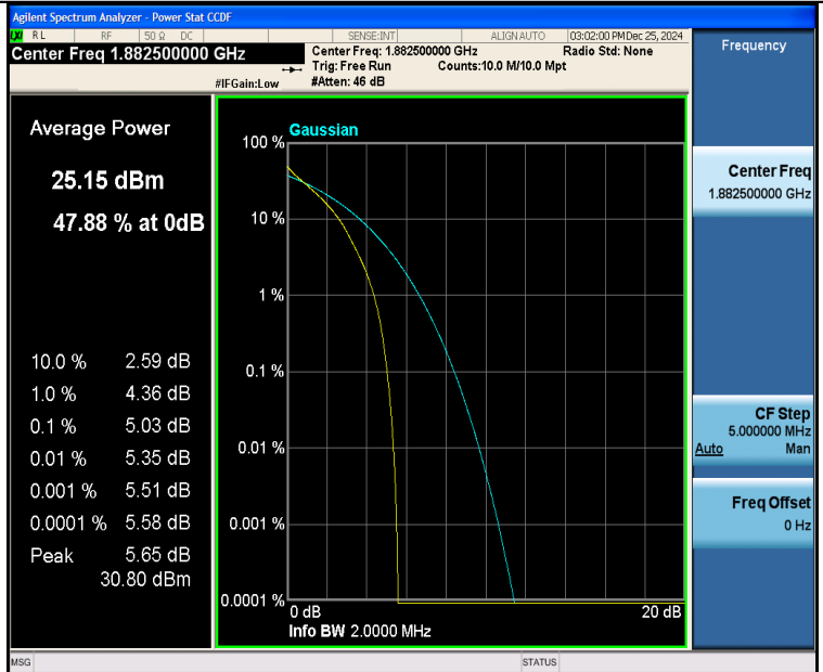
Band25-1.4MHz-QPSK-26365-6RB#0-PASS
