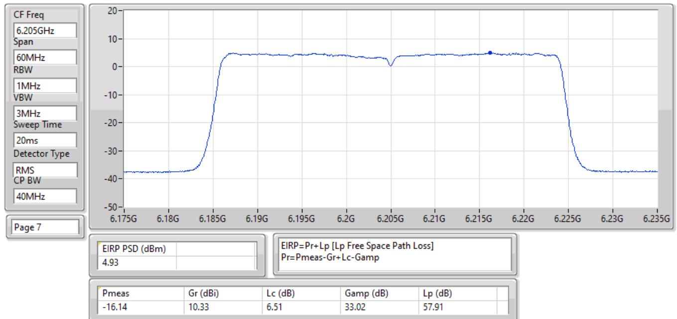
EIRP PSD;Band:6.2G;be40,BF;BWch:40MHz;Nss:2,(M0);Nant:4;Ch:6205MHz;TX
