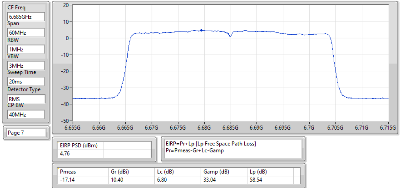
EIRP PSD;Band:6.7G;be40,BF;BWch:40MHz;Nss:2,(M0);Nant:4;Ch:6685MHz;TX
