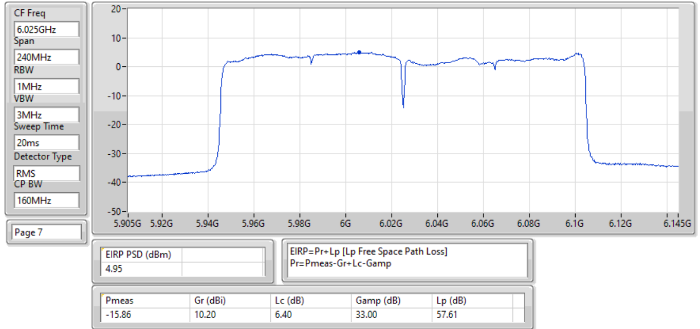
EIRP PSD;Band:6.2G;be160,BF;BWch:160MHz;Nss:2,(M0);Nant:4;Ch:6025MHz;TX
