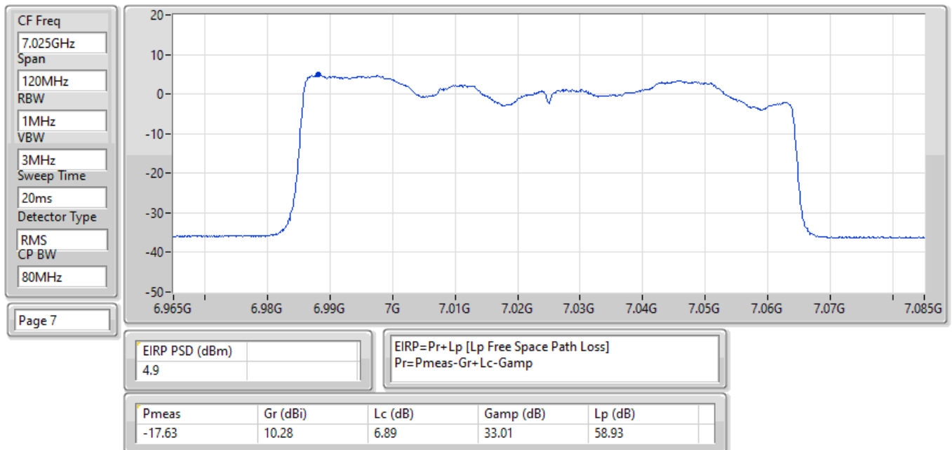
EIRP PSD;Band:7.0G;be80,BF;BWch:80MHz;Nss:2,(M0);Nant:4;Ch:7025MHz;TX
