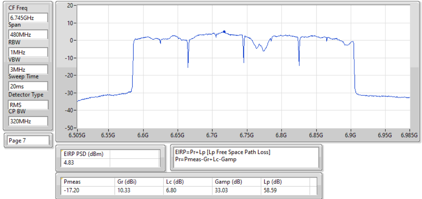
EIRP PSD;Band:6.7G;be320,BF;BWch:320MHz;Nss:2,(M0);Nant:4;Ch:6745MHz;TX
