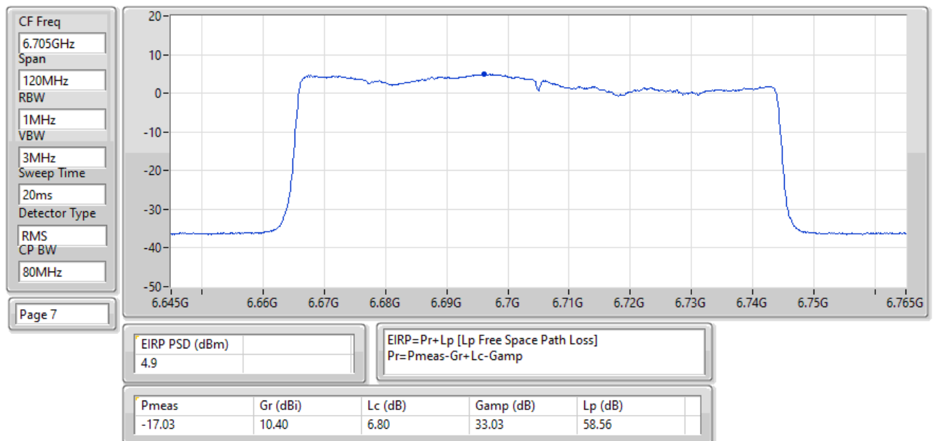
EIRP PSD;Band:6.7G;be80,BF;BWch:80MHz;Nss:2,(M0);Nant:4;Ch:6705MHz;TX
