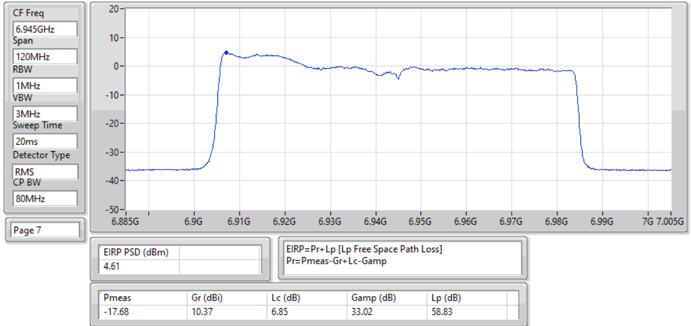
EIRP PSD;Band:7.0G;be80,BF;BWch:80MHz;Nss:2,(M0);Nant:4;Ch:6945MHz;TX
