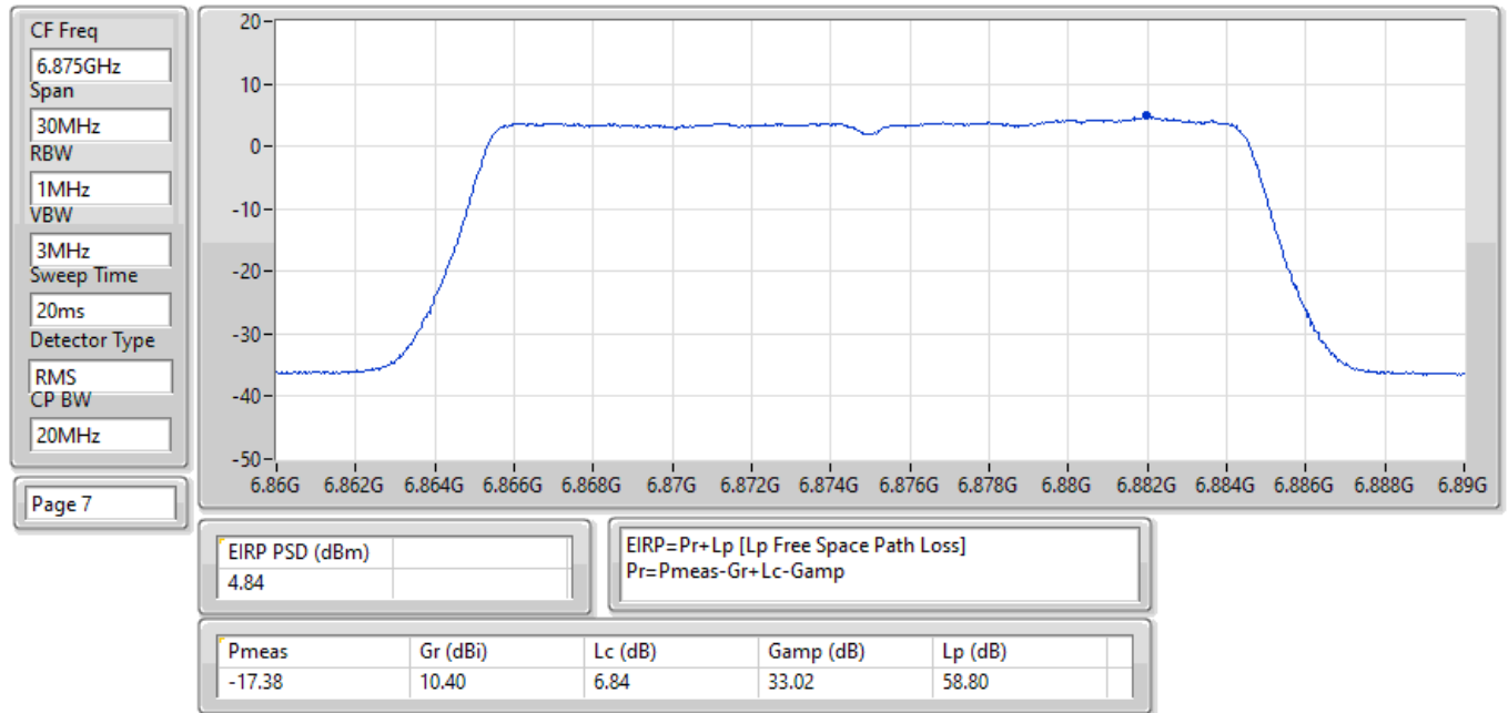
EIRP PSD;Band:6.7G;be20,BF;BWch:20MHz;Nss:2,(M0);Nant:4;Ch:6875MHz;TX
