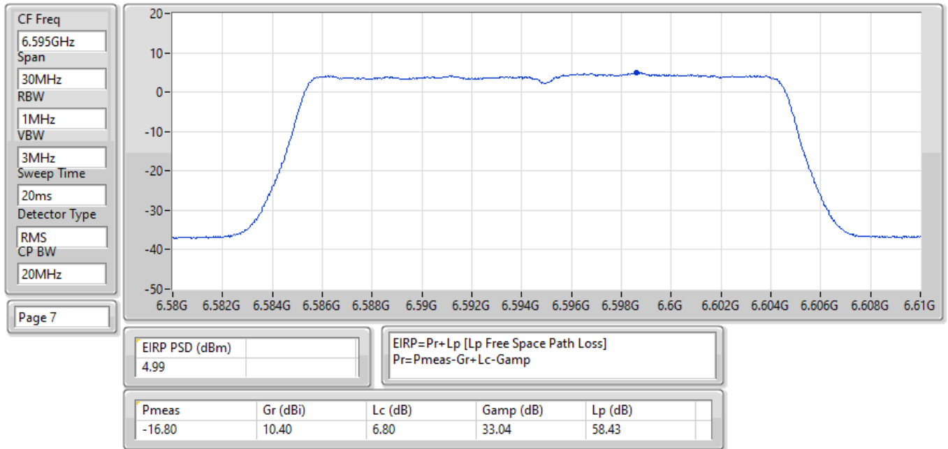
EIRP PSD;Band:6.7G;be20,BF;BWch:20MHz;Nss:2,(M0);Nant:4;Ch:6595MHz;TX
