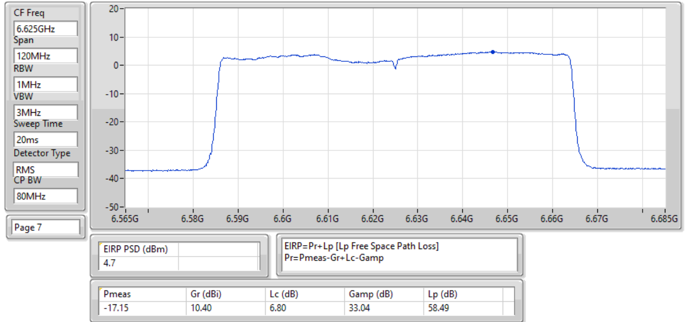
EIRP PSD;Band:6.7G;be80,BF;BWch:80MHz;Nss:2,(M0);Nant:4;Ch:6625MHz;TX
