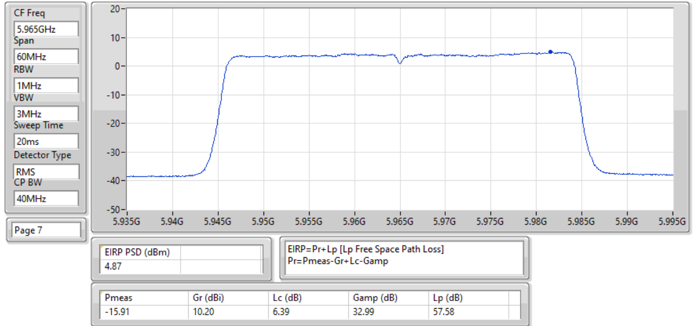
EIRP PSD;Band:6.2G;be40,BF;BWch:40MHz;Nss:2,(M0);Nant:4;Ch:5965MHz;TX
