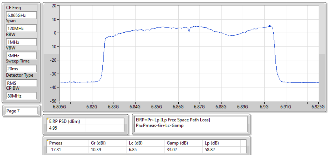
EIRP PSD;Band:6.7G;be80,BF;BWch:80MHz;Nss:2,(M0);Nant:4;Ch:6865MHz;TX
