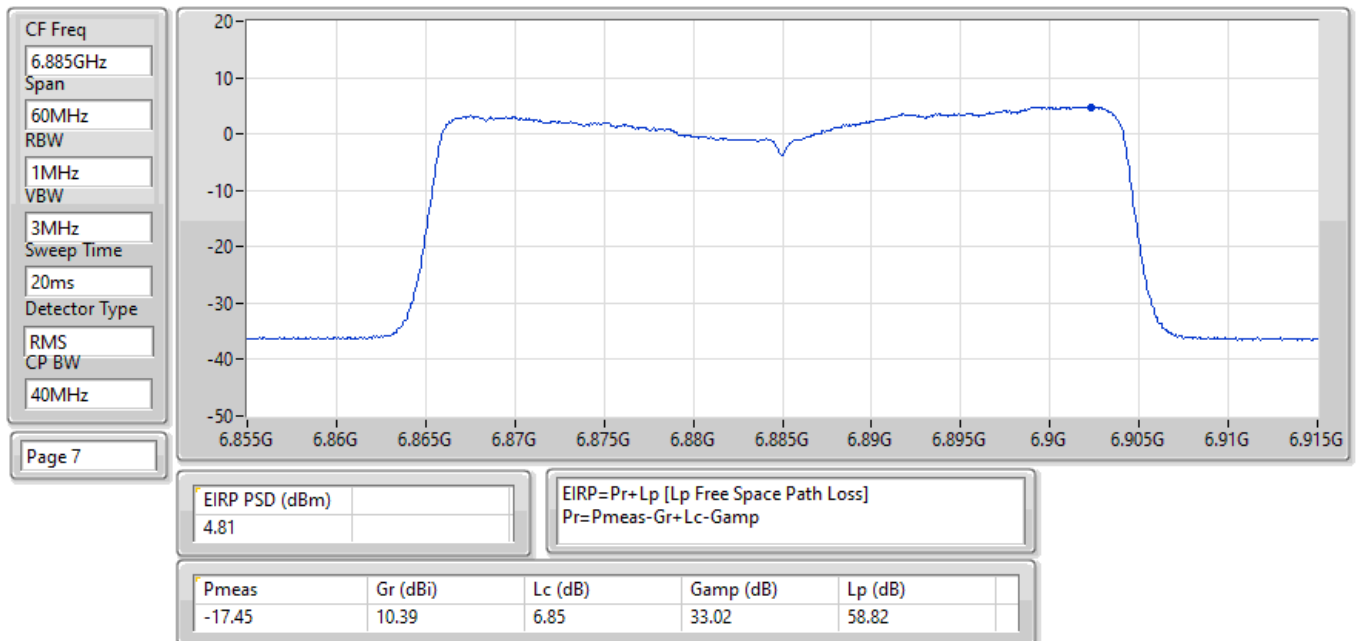
EIRP PSD;Band:6.7G;be40,BF;BWch:40MHz;Nss:2,(M0);Nant:4;Ch:6885MHz;TX
