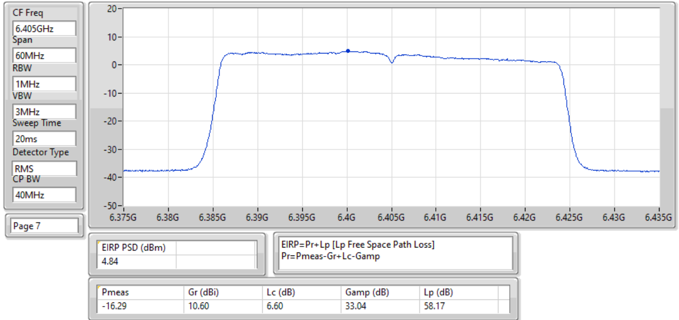
EIRP PSD;Band:6.2G;be40,BF;BWch:40MHz;Nss:2,(M0);Nant:4;Ch:6405MHz;TX
