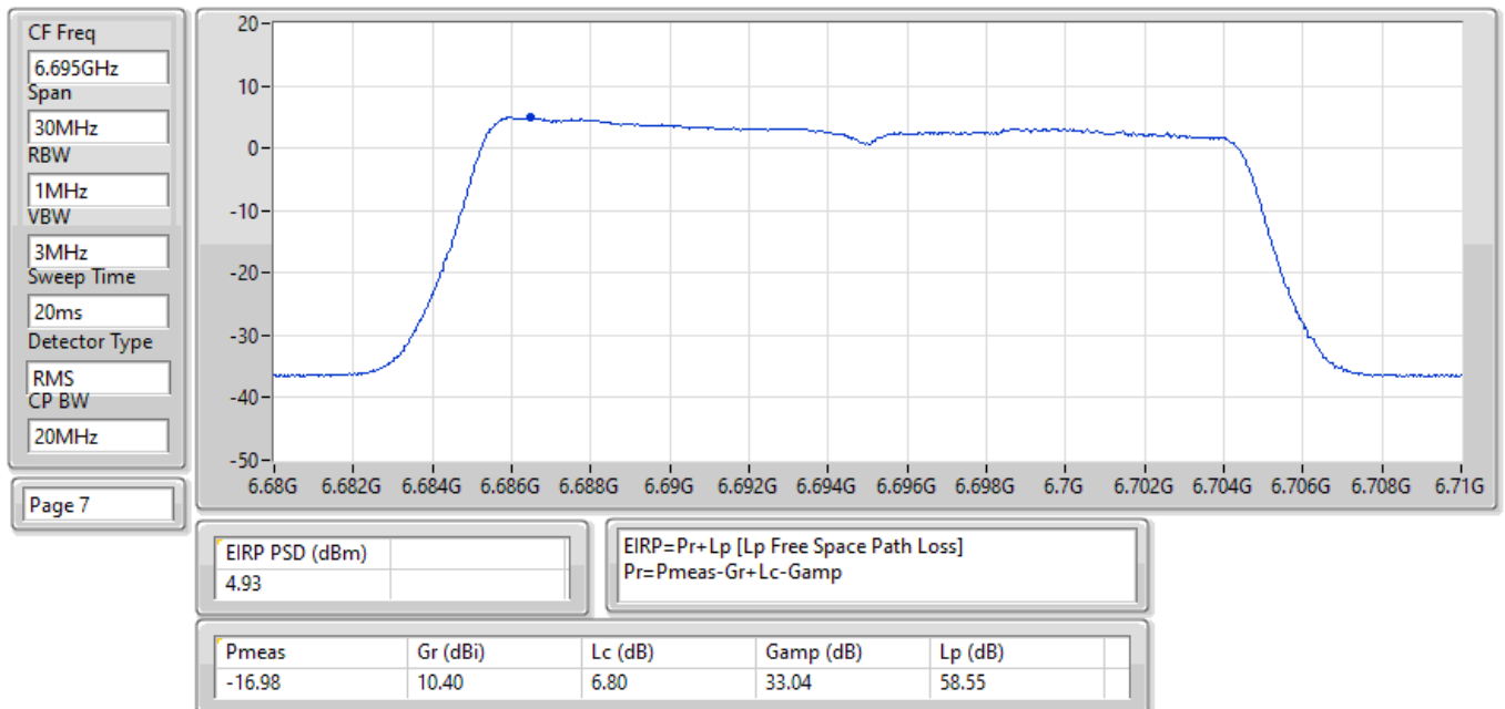
EIRP PSD;Band:6.7G;be20,BF;BWch:20MHz;Nss:2,(M0);Nant:4;Ch:6695MHz;TX
