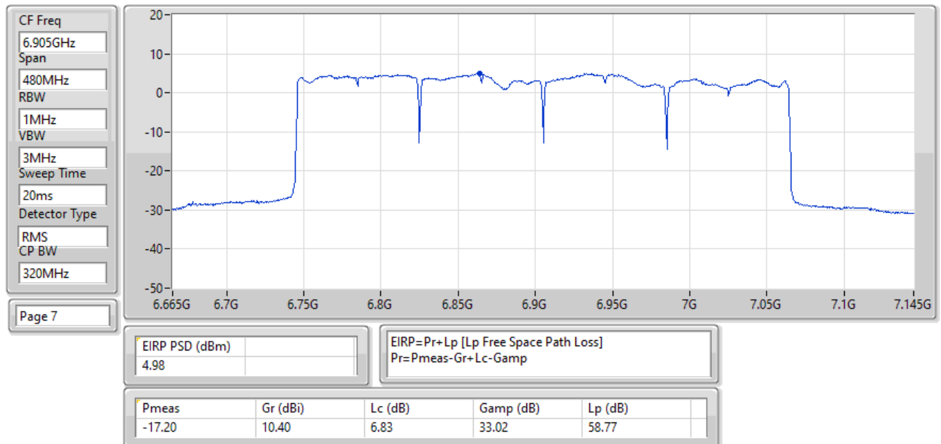
EIRP PSD;Band:7.0G;be320,BF;BWch:320MHz;Nss:2,(M0);Nant:4;Ch:6905MHz;TX
