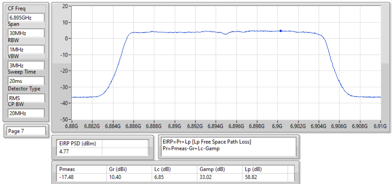
EIRP PSD;Band:7.0G;be20,BF;BWch:20MHz;Nss:2,(M0);Nant:4;Ch:6895MHz;TX
