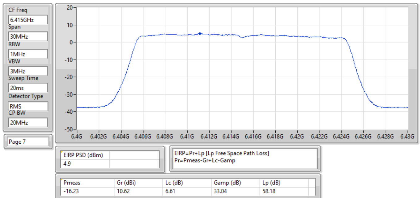
EIRP PSD;Band:6.2G;be20,BF;BWch:20MHz;Nss:2,(M0);Nant:4;Ch:6415MHz;TX
