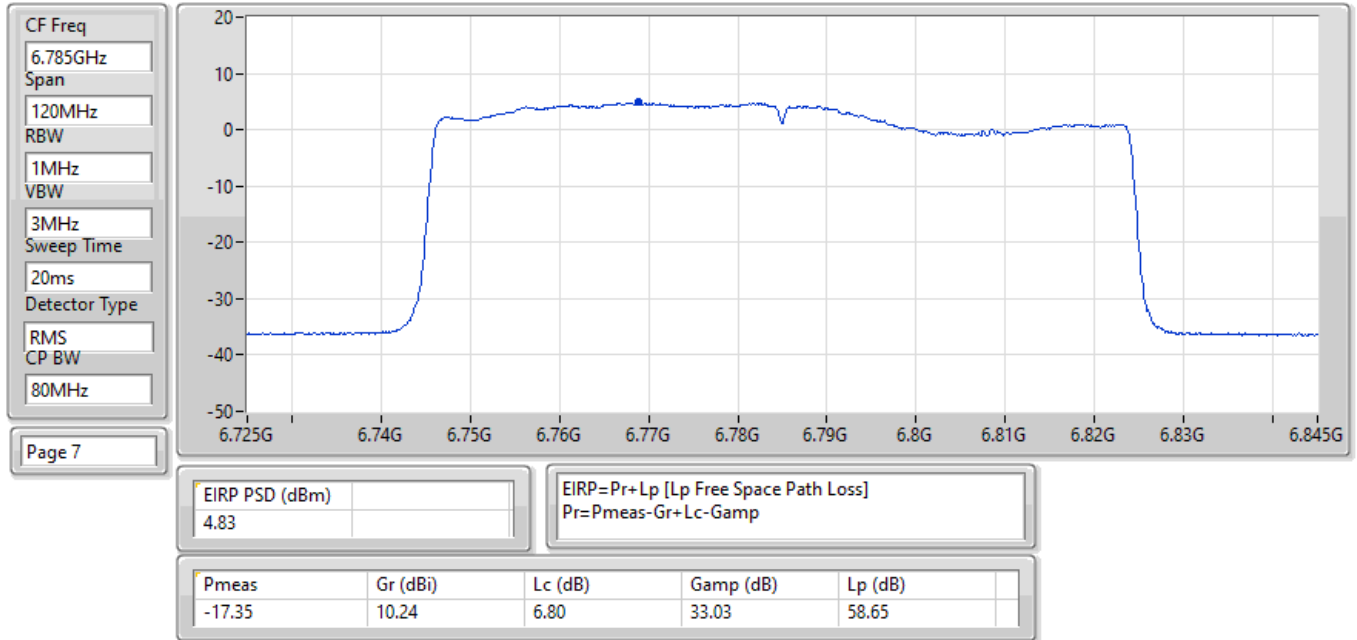
EIRP PSD;Band:6.7G;be80,BF;BWch:80MHz;Nss:2,(M0);Nant:4;Ch:6785MHz;TX
