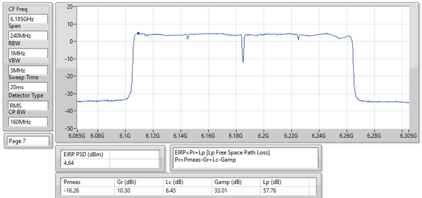
EIRP PSD;Band:6.2G;be160,BF;BWch:160MHz;Nss:2,(M0);Nant:4;Ch:6185MHz;TX
