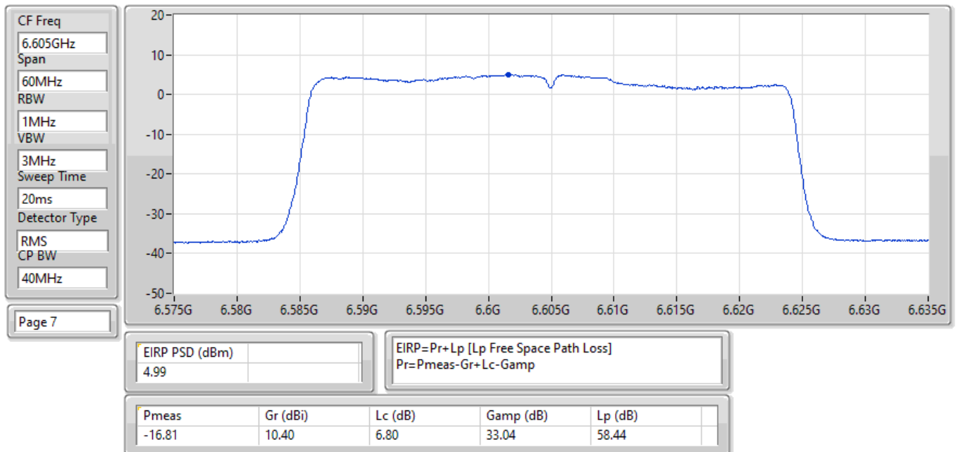
EIRP PSD;Band:6.7G;be40,BF;BWch:40MHz;Nss:2,(M0);Nant:4;Ch:6605MHz;TX
