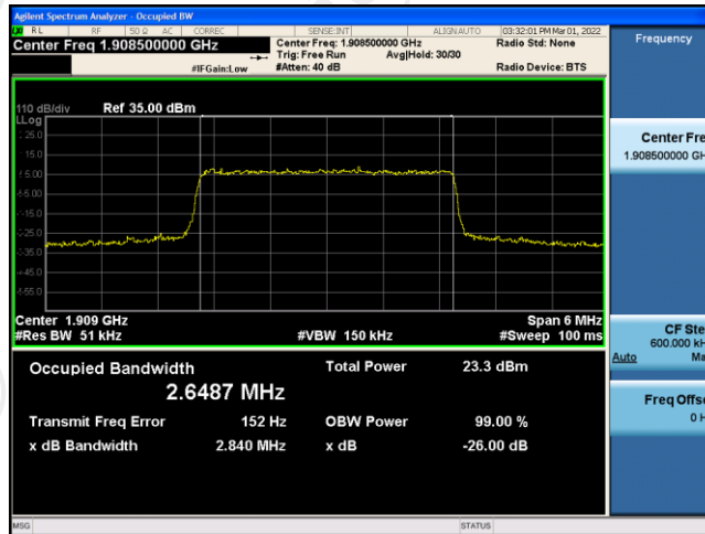
Band2-3MHz-16QAM-18615-15RB#0
