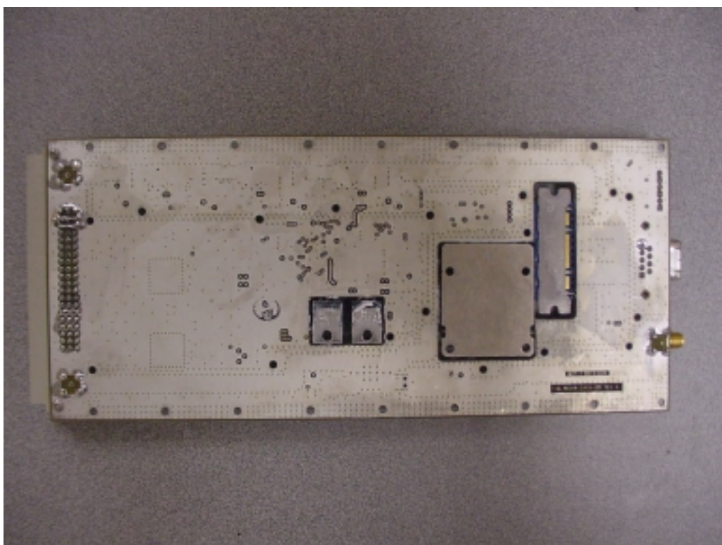
800 MHz Amplifier Module - Bottom
