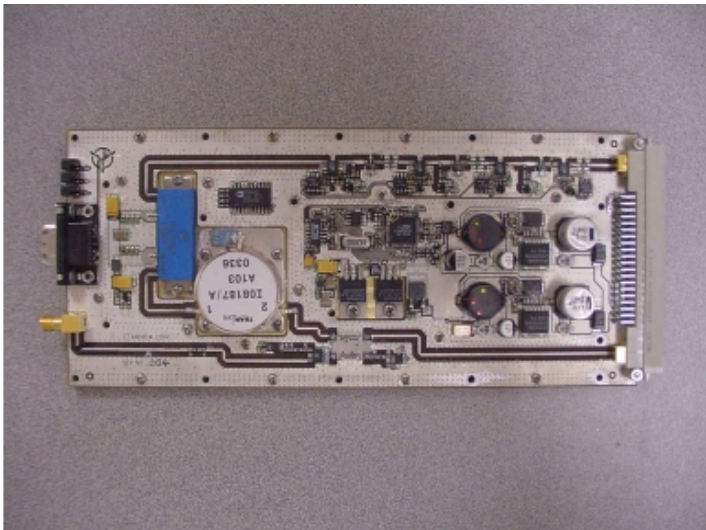
800 MHz Amplifier Module - Top
