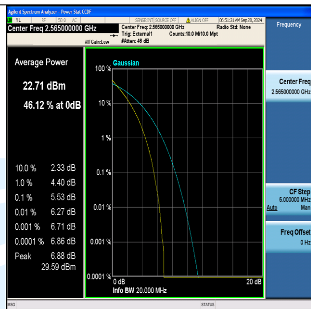
Band41(2555-2655)-20MHz-QPSK-40340-100RB#0-PASS
