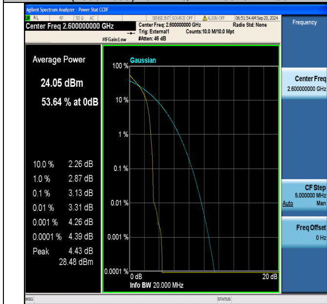
Band41(2555-2655)-20MHz-QPSK-40690-1RB#0-PASS
