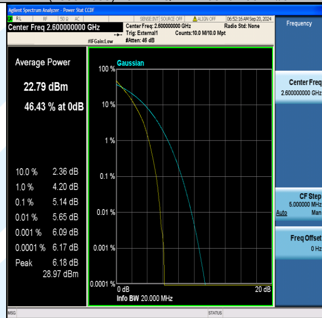
Band41(2555-2655)-20MHz-QPSK-40690-100RB#0-PASS
