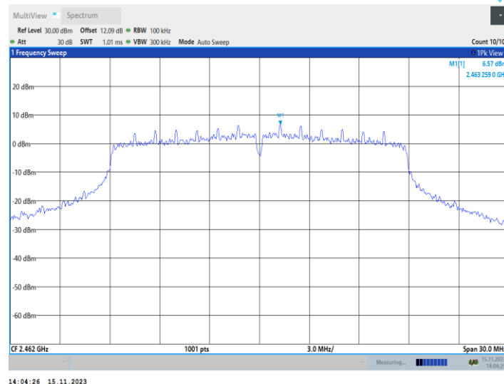
11N20MIMO Ant1 2462 30-1000
