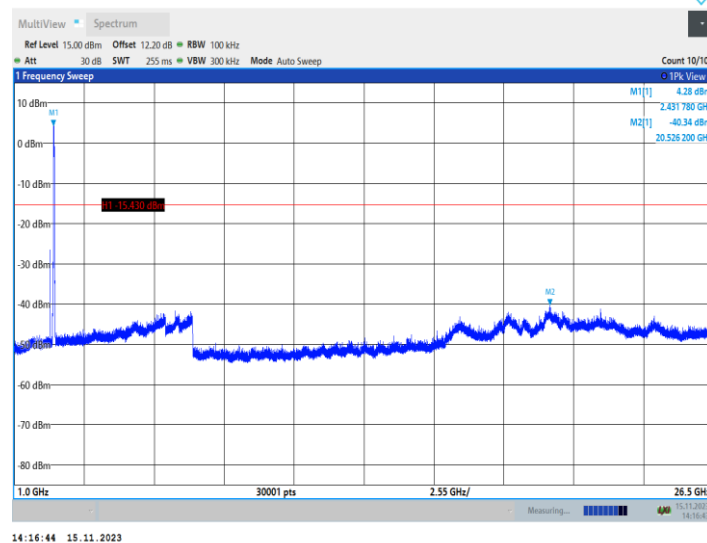
11N40MIMO_Ant1_2452_0-Reference
