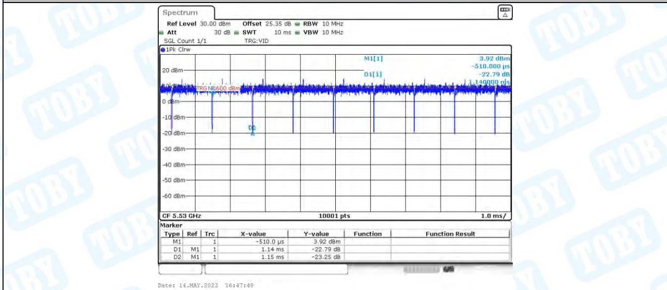
11AC80MIMO_Ant4_5530
