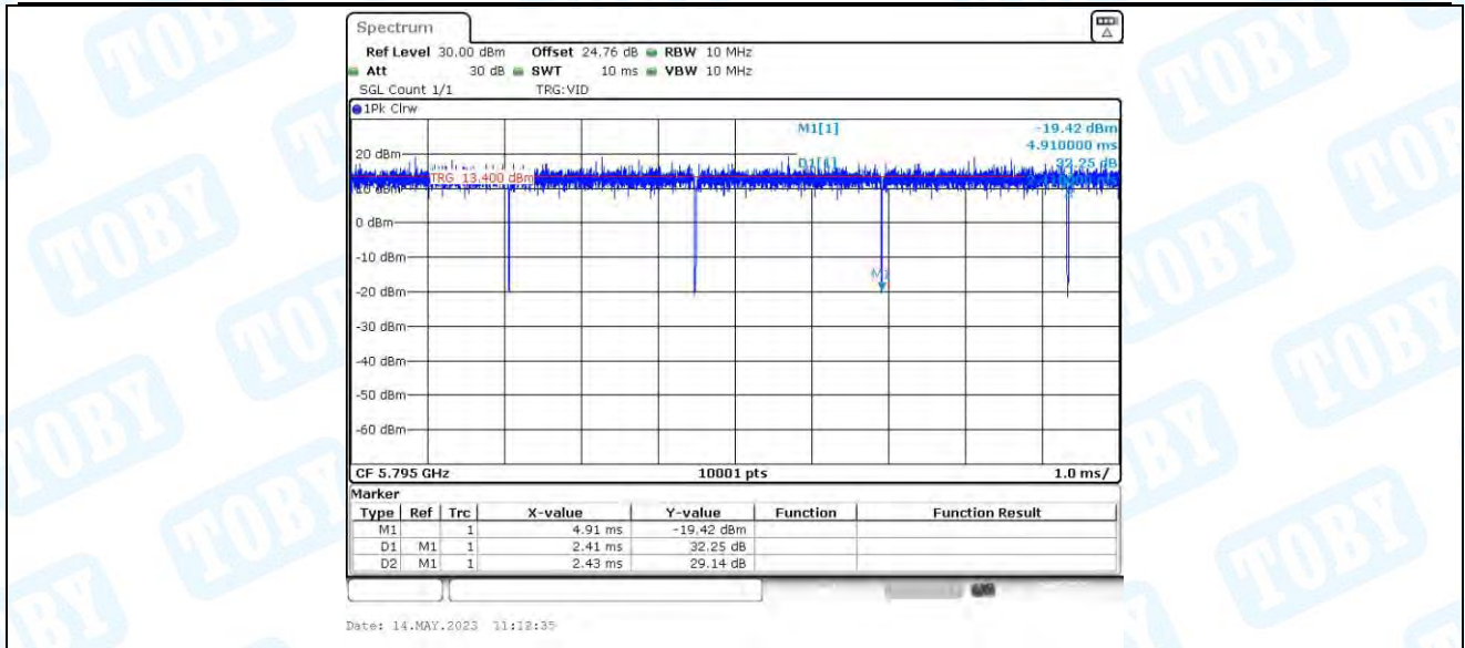
11N40MIMO_Ant2_5795
