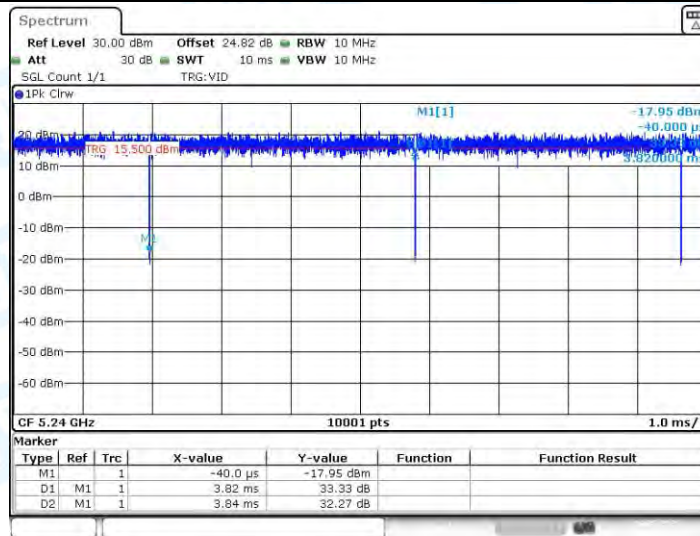
11AX20MIMO_Ant4_5240
