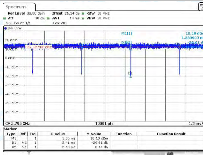
11AC40MIMO_Ant4_5795
