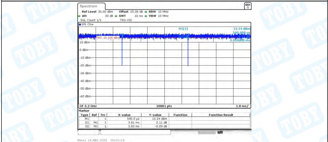
11AX20MIMO_Ant3_5200
