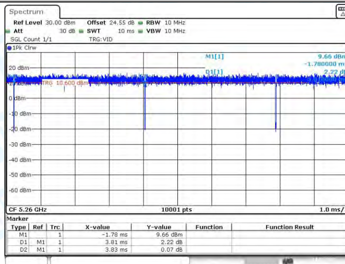
11AX20MIMO_Ant1_5260
