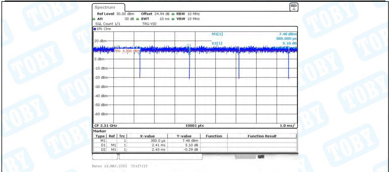
11AC40MIMO_Ant2_5510
