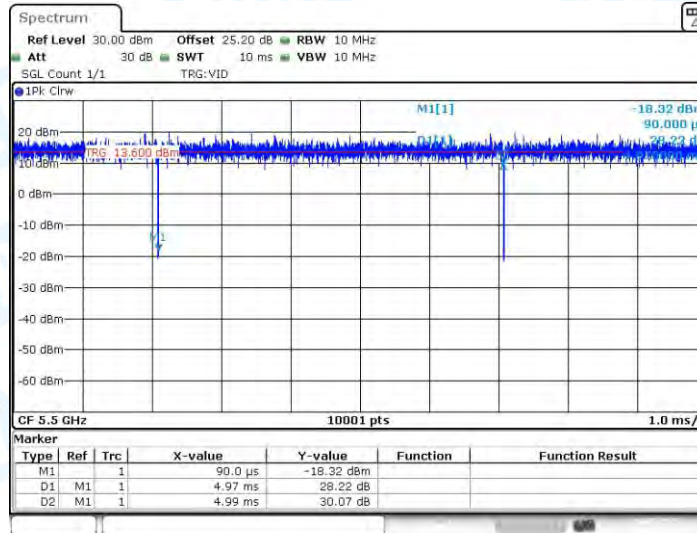
11AC20MIMO_Ant4_5500
