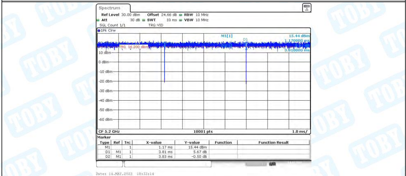
11AX20MIMO_Ant4_5200
