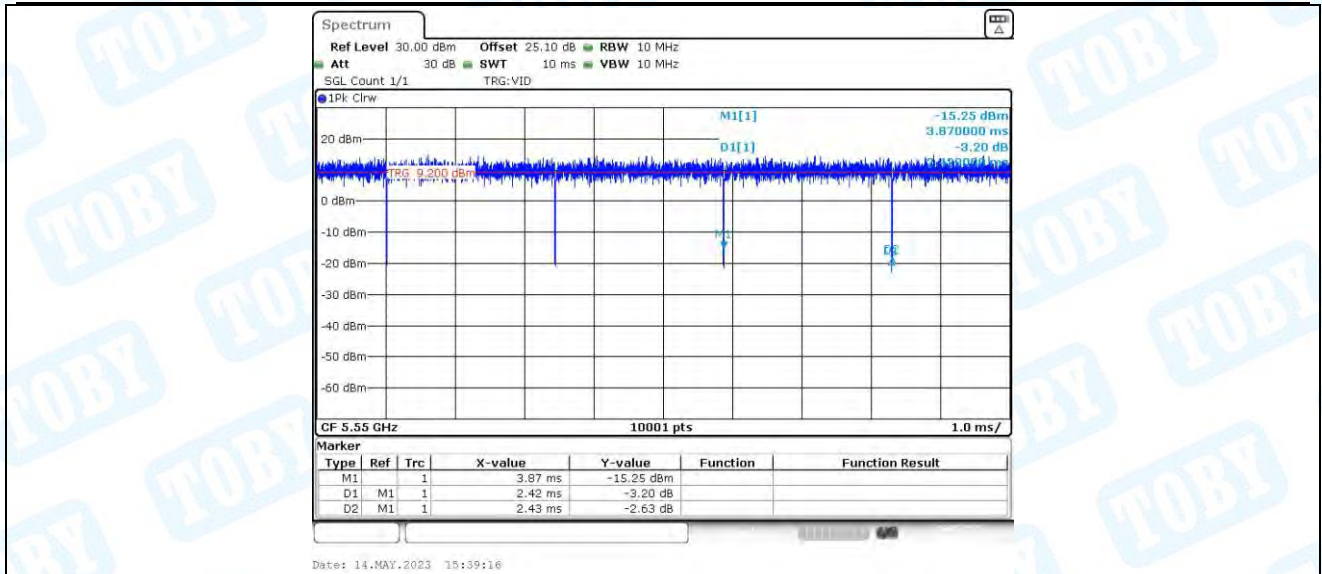
11AC40MIMO_Ant4_5550
