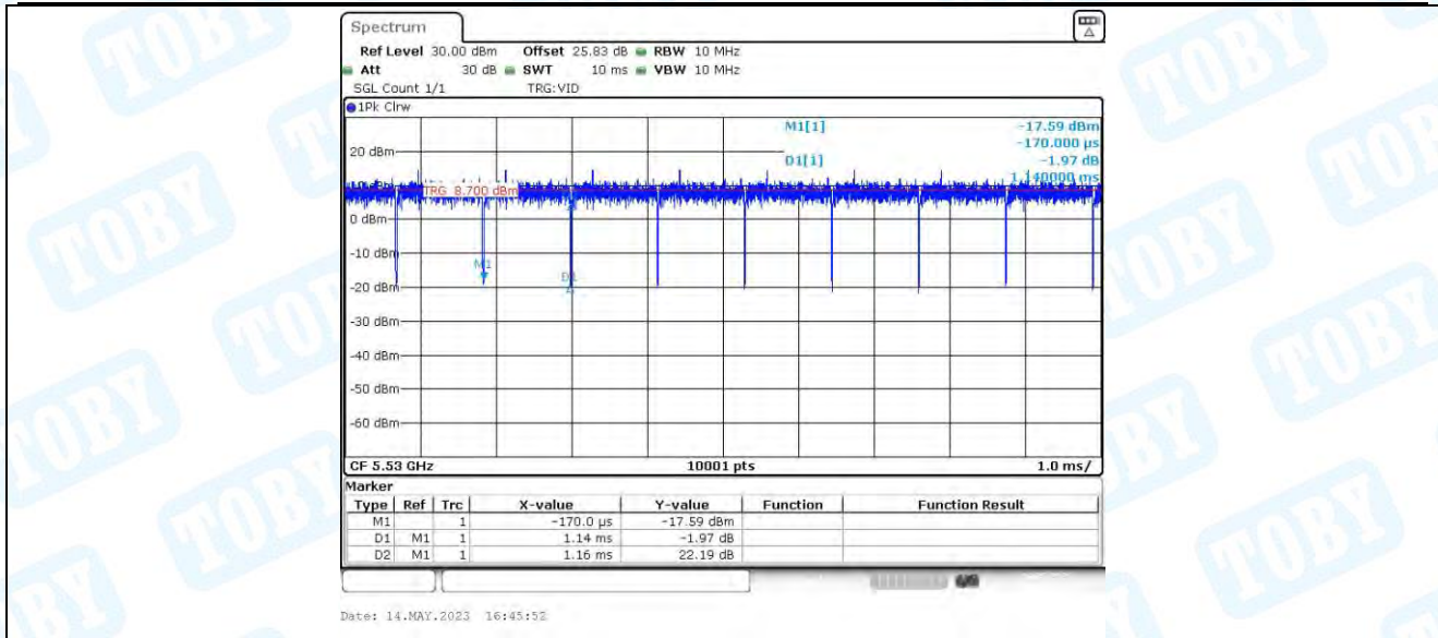
11AC80MIMO_Ant3_5530
