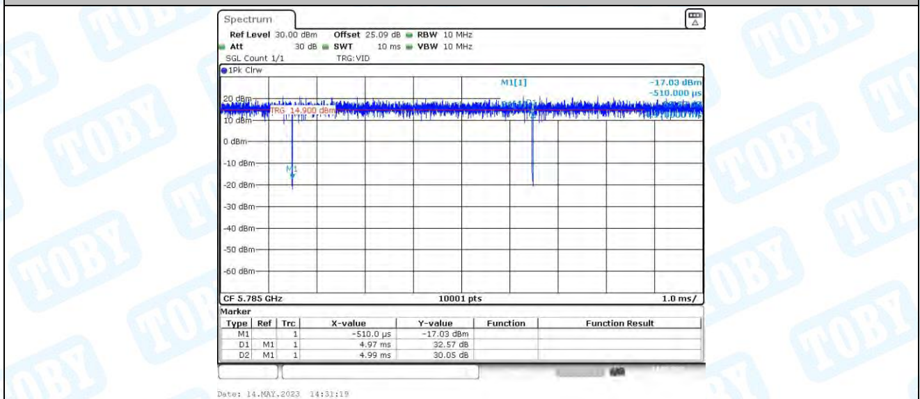
11AC20MIMO_Ant4_5785
