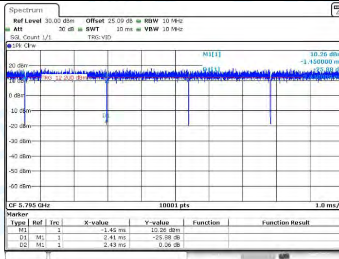
11AC40MIMO_Ant3_5795
