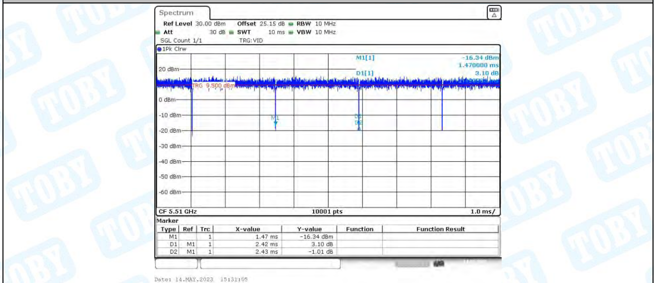
11AC40MIMO_Ant4_5510
