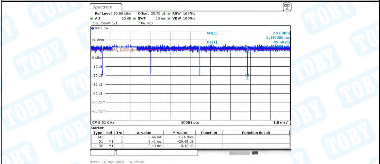
11AC40MIMO_Ant3_5510
