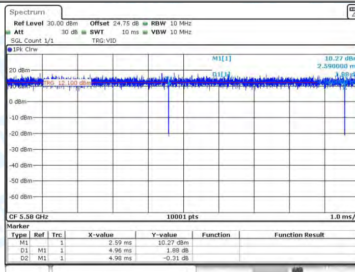
11AC20MIMO_Ant1_5580
