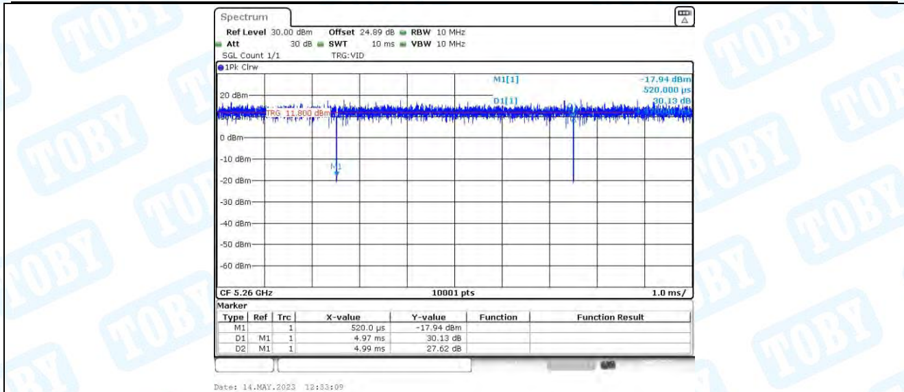
11AC20MIMO_Ant4_5260
