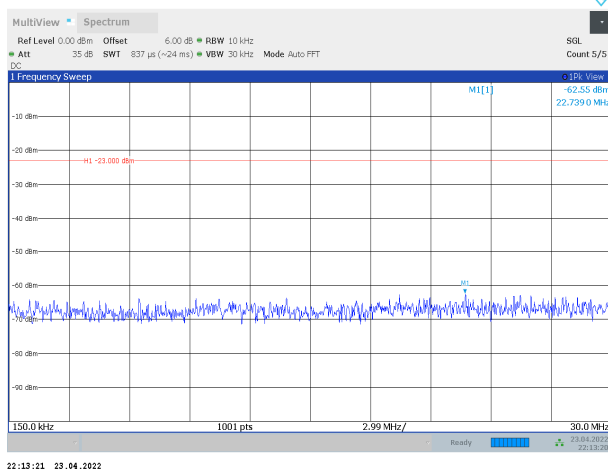
Band43-20MHz-QPSK-44690-1RB#0-Range2:0.15~30MHz
