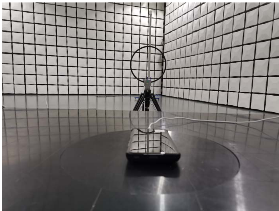
9KHz~30MHz
