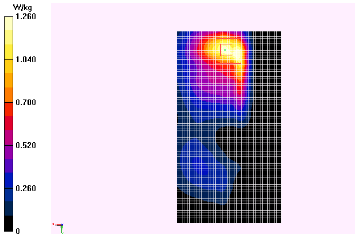
Fig.8 WCDMA1900 CH9400
