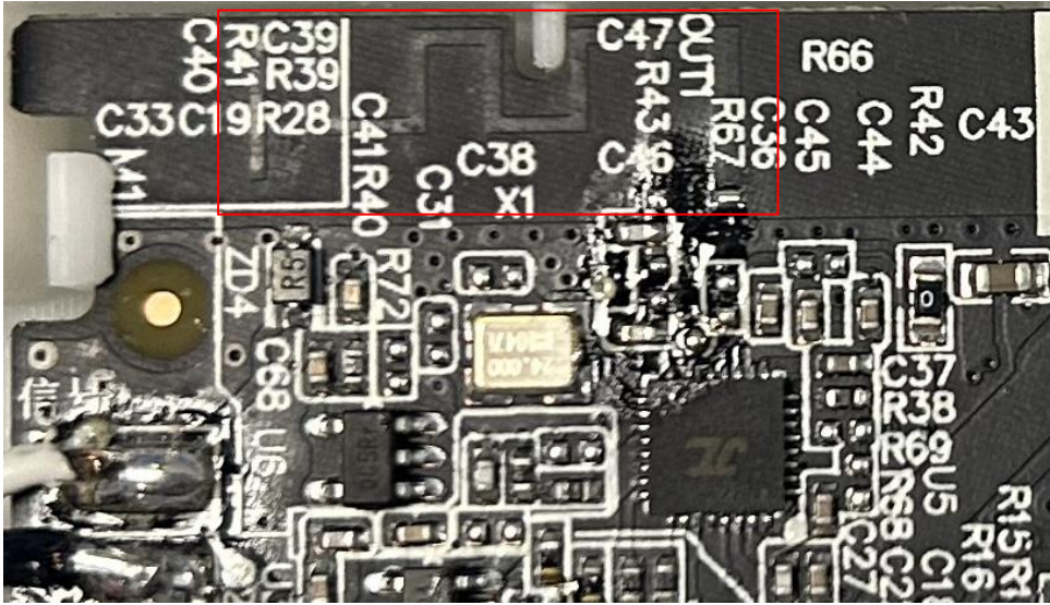
BLE Antenna
