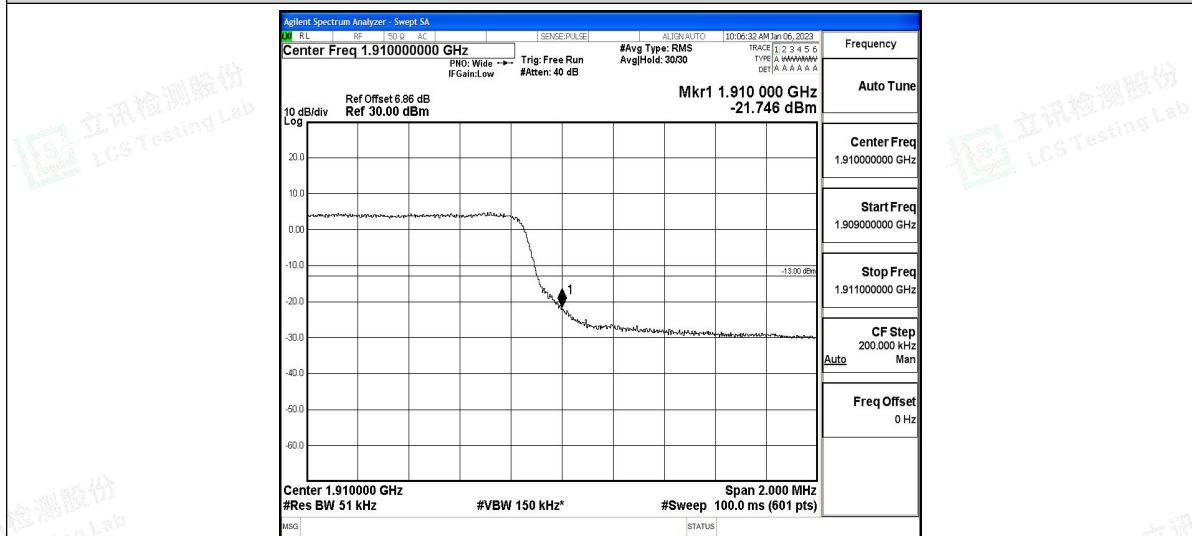
Band2-3MHz-16QAM-18615-15RB#0
