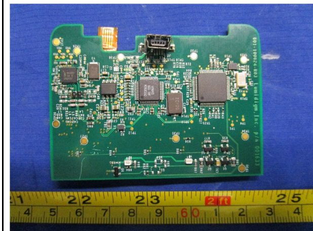
PCBA 2 Bottom View2
