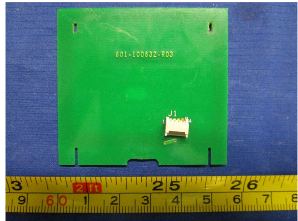
PCBA 2(ANTENNA) Bottom View3
