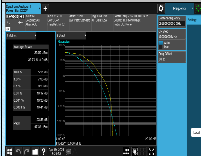
41(2535-2655)-10MHz-QPSK-41190-1RB#0-PASS
