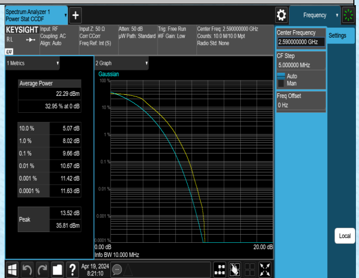
41(2535-2655)-10MHz-QPSK-40590-50RB#0-PASS
