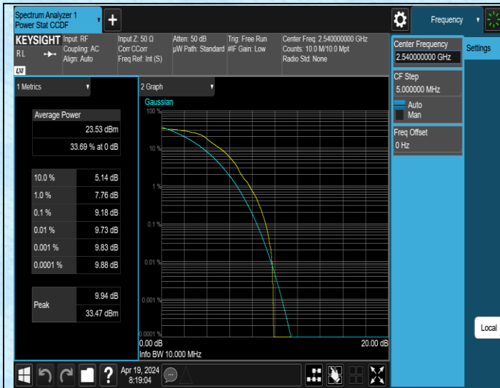
41(2535-2655)-10MHz-QPSK-40090-1RB#0-PASS
