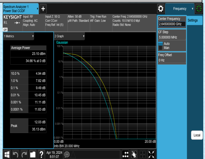
41(2535-2655)-20MHz-QPSK-41140-100RB#0-PASS
