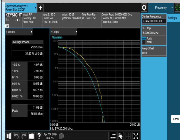
41(2535-2655)-20MHz-QPSK-41140-1RB#0-PASS
