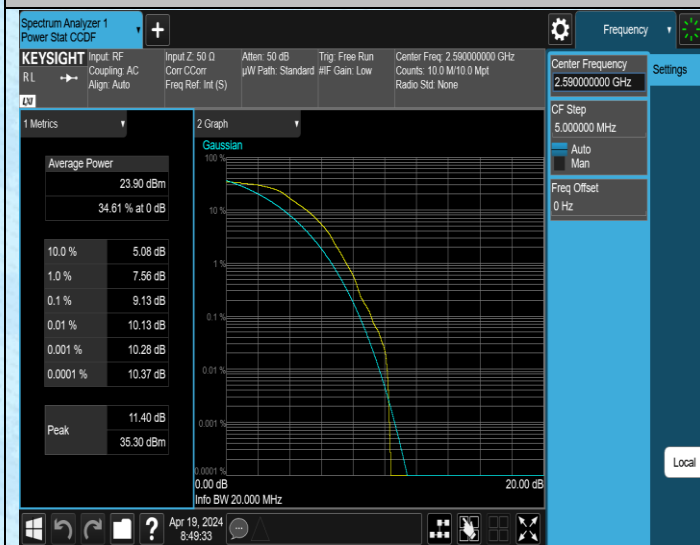
41(2535-2655)-20MHz-QPSK-40590-1RB#0-PASS
