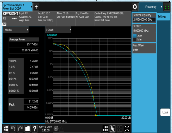
41(2535-2655)-20MHz-QPSK-40140-100RB#0-PASS
