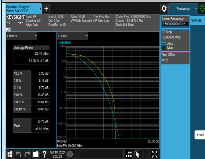
41(2535-2655)-10MHz-QPSK-40590-1RB#0-PASS
