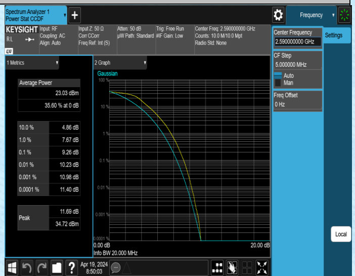
41(2535-2655)-20MHz-QPSK-40590-100RB#0-PASS
