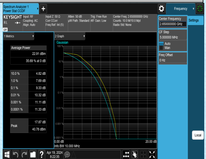
41(2535-2655)-10MHz-QPSK-41190-50RB#0-PASS
