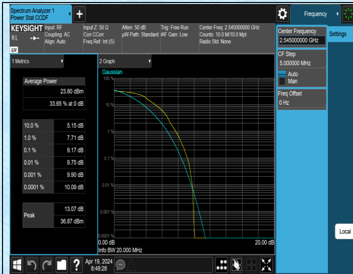
41(2535-2655)-20MHz-QPSK-40140-1RB#0-PASS
