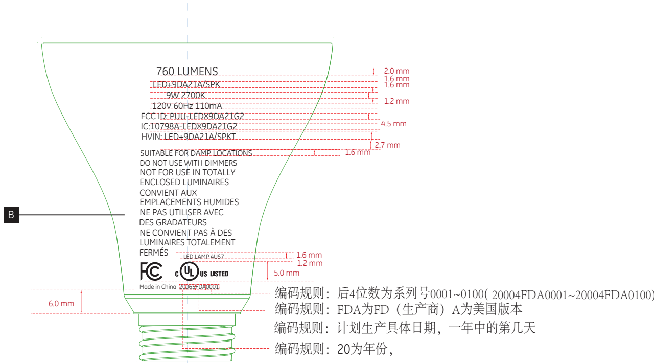
LED灯9A2700K 版本（背面）
