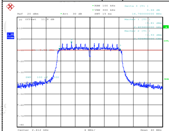
802.11n(HT20)
