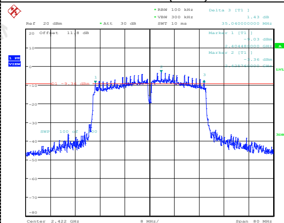
802.11n(HT40)
