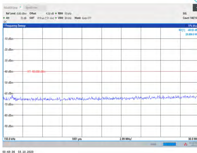
Band48-20MHz-QPSK-55340-1RB#0-Range2:0.15~30MHz
