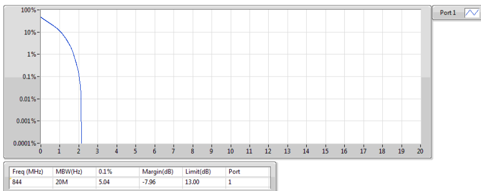
Band 26_LTE-M1_10MHz_Nss1,QPSK_1TX 844MHz_QPSK_RB 6,#RB 0,NB 7
