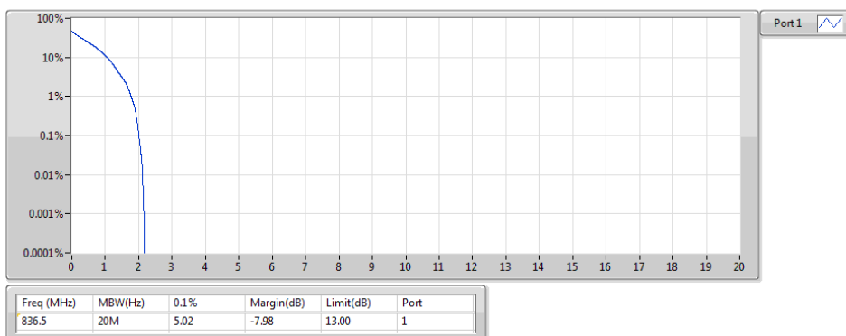
Band 26_LTE-M1_10MHz_Nss1,QPSK_1TX 836.5MHz_QPSK_RB 6,#RB 0,NB 0
