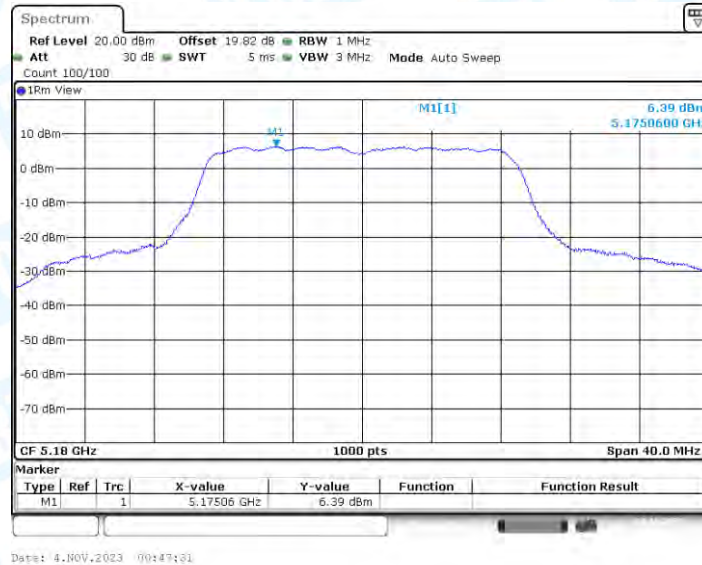
11N20-BF_Ant2_5180
