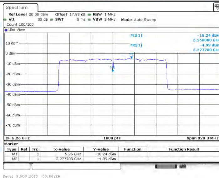
11AX160-CDD_Ant3_5250_UNII-2A
