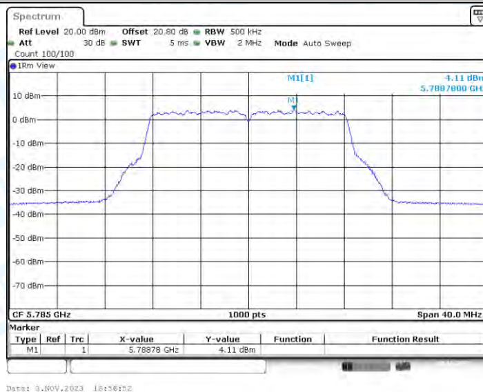
11A-BF_Ant4_5785
