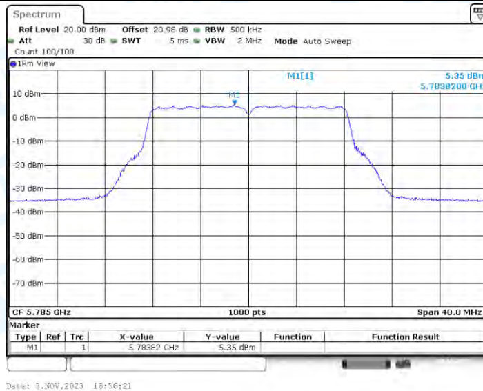
11A-BF_Ant3_5785
