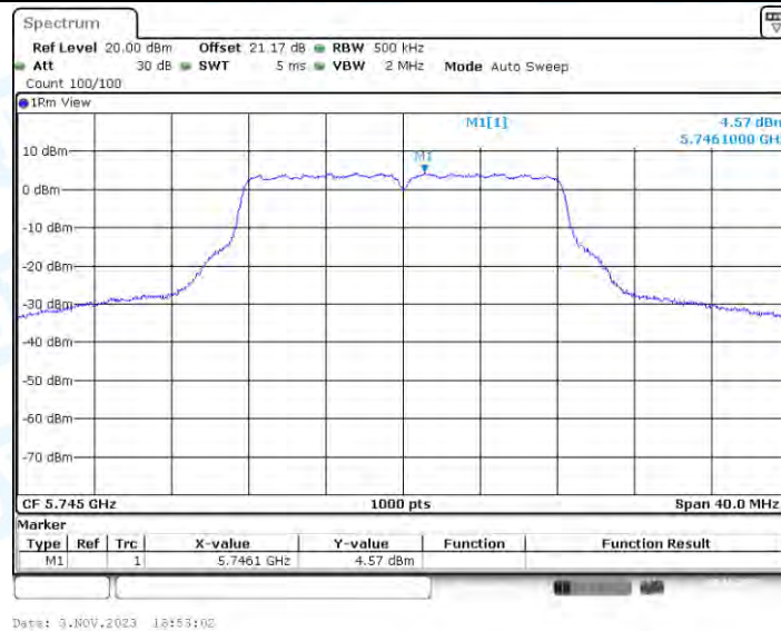
11A-BF_Ant4_5745
