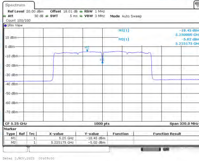
11AX160-CDD_Ant1_5250_UNII-2A
