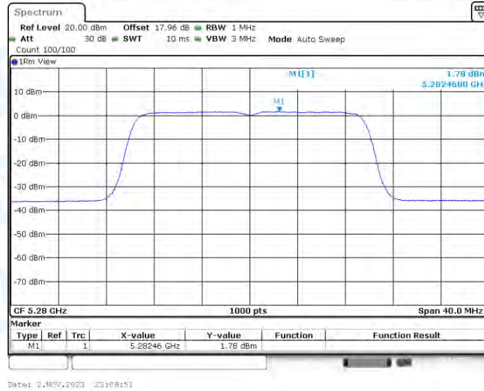
11AX20-CDD_Ant3_5280
