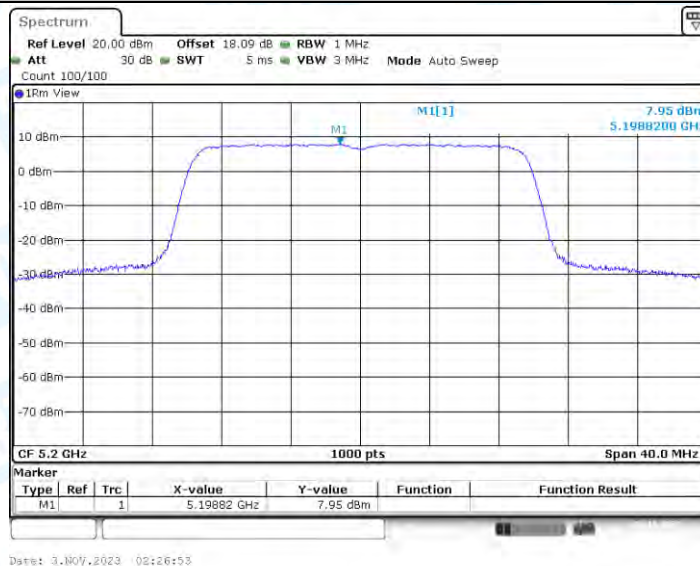
11AX20-CDD_Ant2_5200
