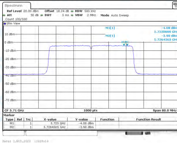
11AX40-CDD_Ant1_5755
