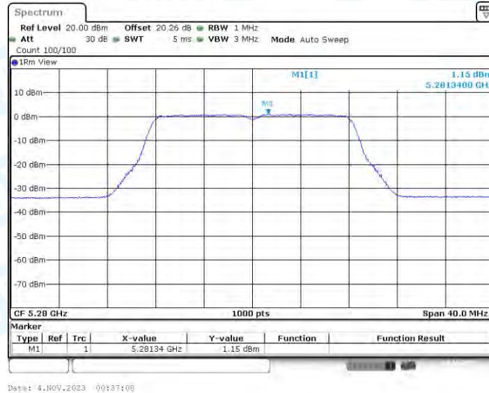
11A-BF_Ant2_5280
