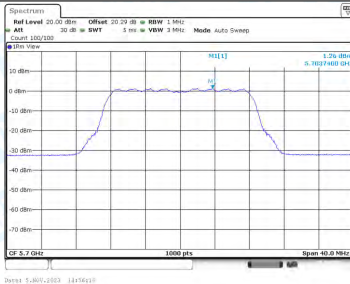
11A-BF_Ant2_5700
