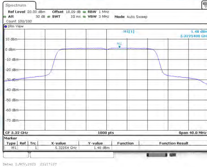
11AX20-CDD_Ant2_5320
