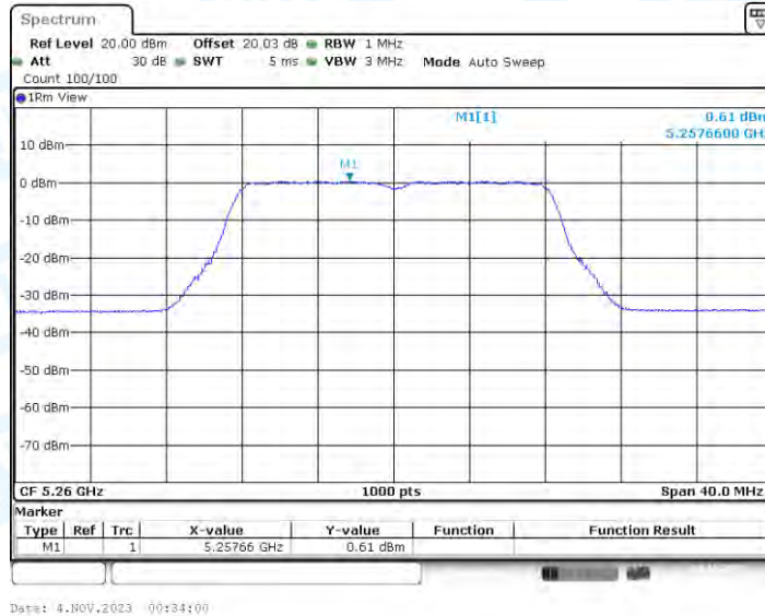
11A-BF_Ant3_5260
