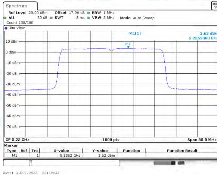
11AX40-CDD_Ant3_5230
