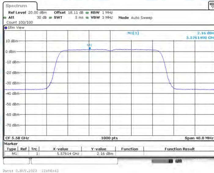
11AX20-CDD_Ant2_5580
