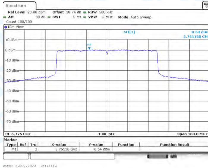
11AX80-CDD_Ant2_5775
