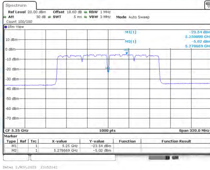
11AC160-CDD_Ant3_5250_UNII-2A
