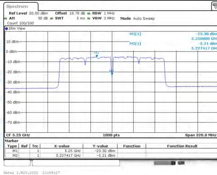
11AC160-CDD_Ant1_5250_UNII-2A
