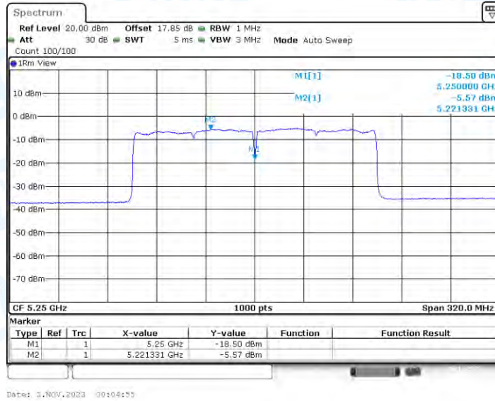
11AX160-CDD_Ant2_5250_UNII-1
