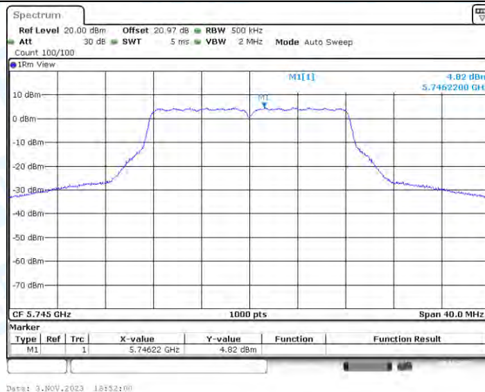
11A-BF_Ant2_5745
