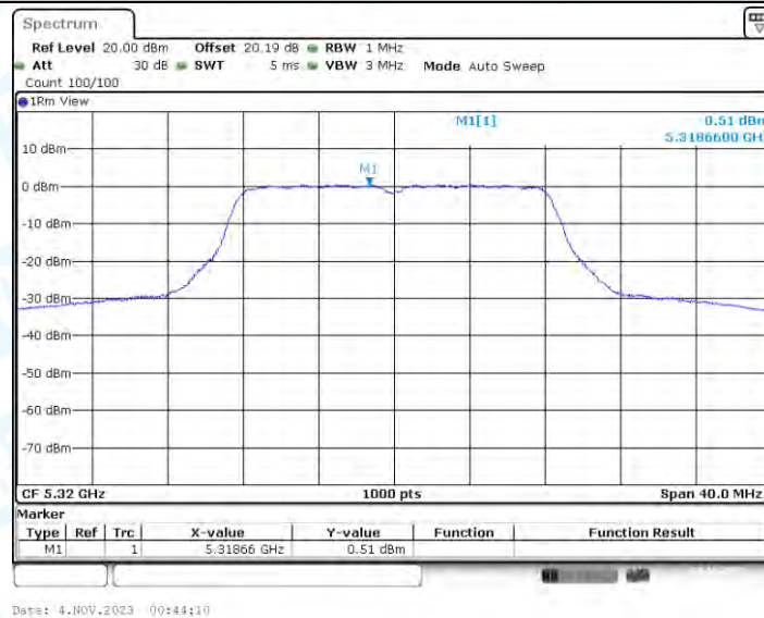
11A-BF_Ant2_5320
