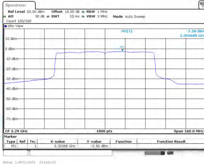
11AX80-CDD_Ant2_5290
