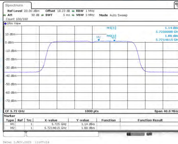
11AX20-CDD_Ant1_5720_UNII-3
