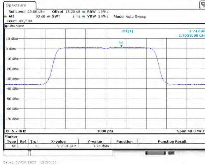
11AX20-CDD_Ant2_5700
