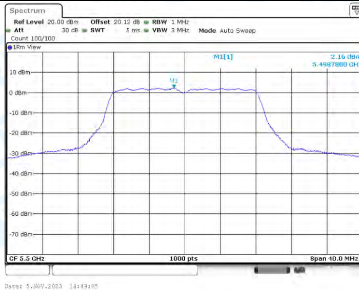
11A-BF_Ant3_5500
