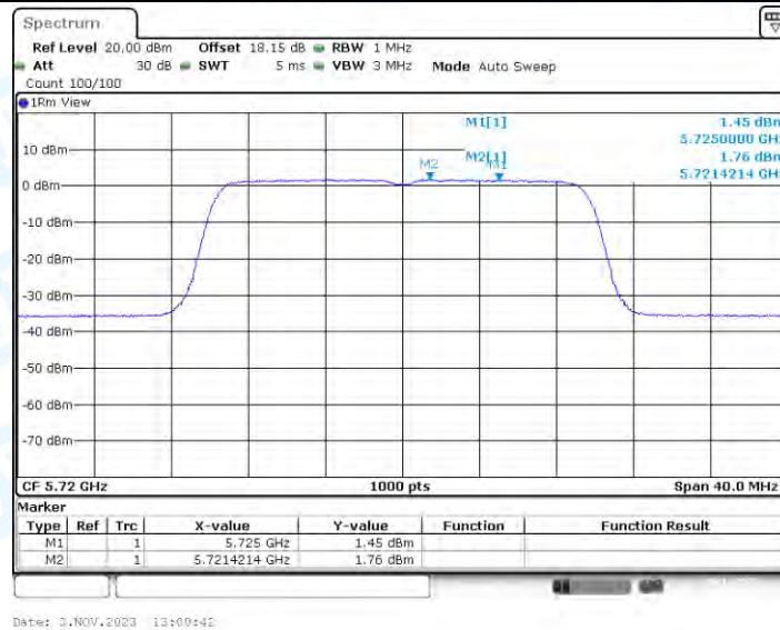
11AX20-CDD_Ant2_5720_UNII-2C
