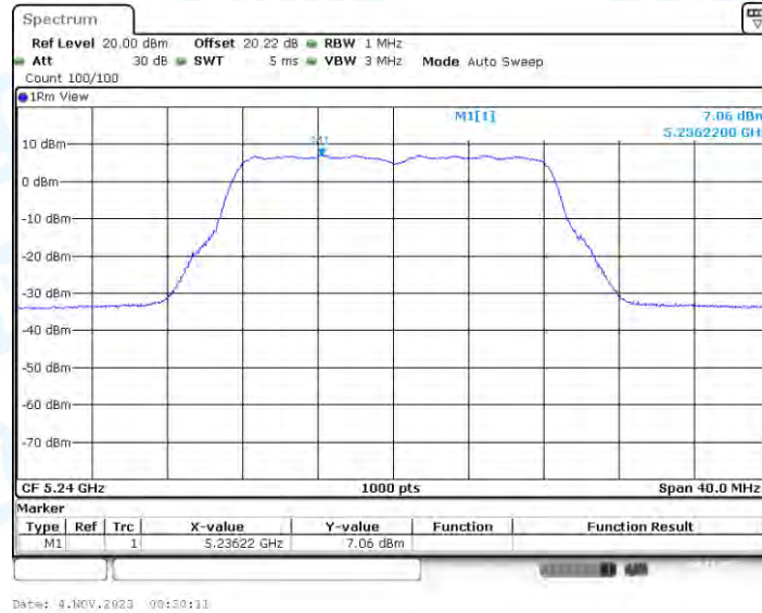
11A-BF_Ant3_5240
