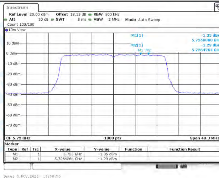
11AX20-CDD_Ant2_5720_UNII-3
