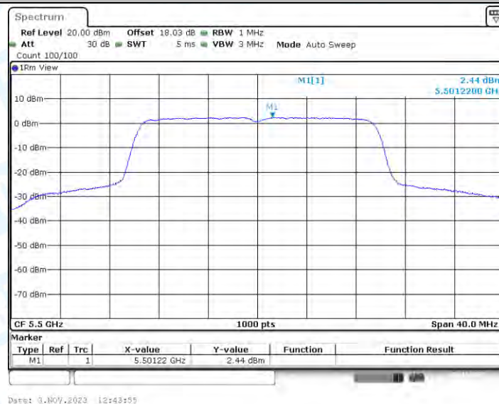
11AX20-CDD_Ant3_5500
