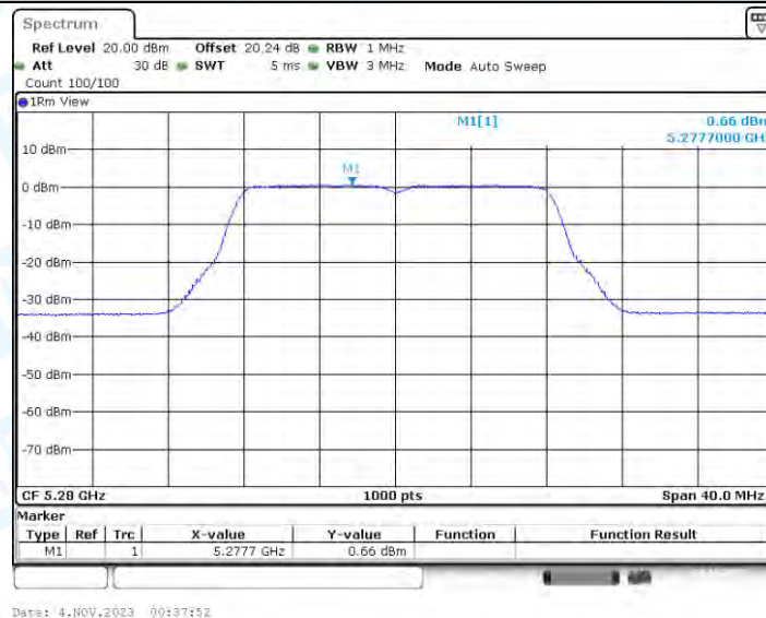
11A-BF_Ant3_5280
