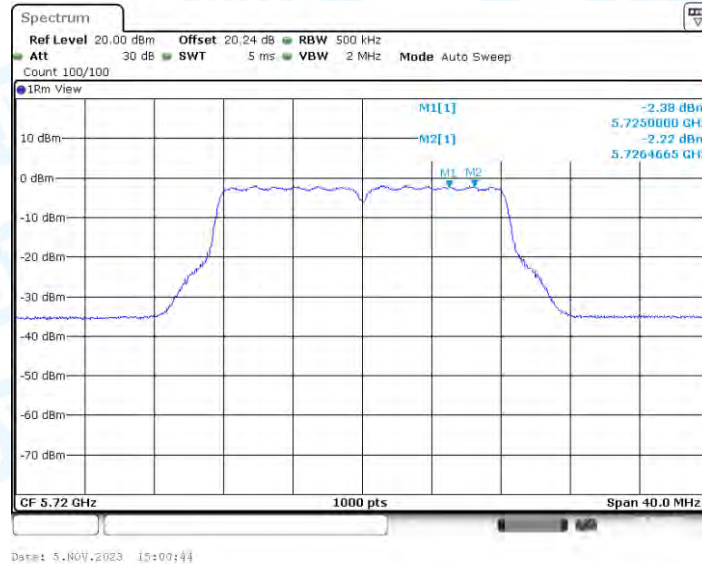
11A-BF_Ant2_5720_UNII-3
