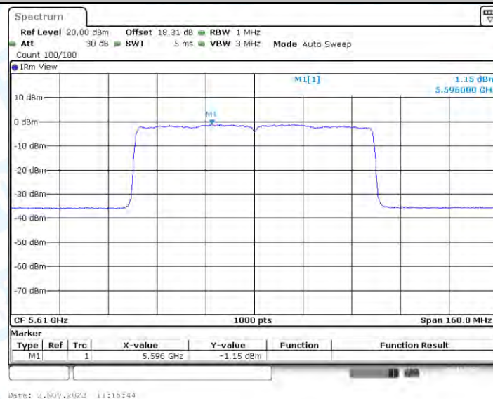
11AX80-CDD_Ant2_5610
