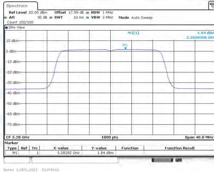
11AX20-CDD_Ant2_5280
