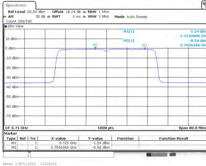
11AX40-CDD_Ant1_5710_UNII-3
