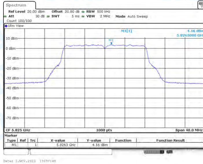
11A-BF_Ant4_5825
