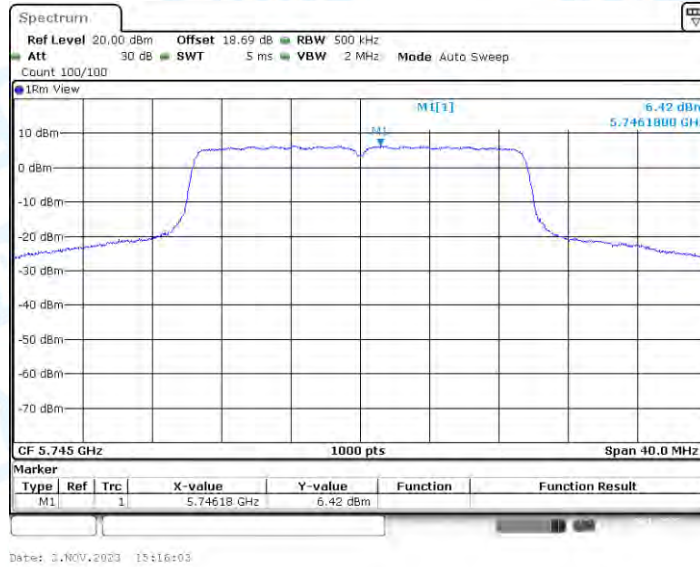
11AX20-CDD_Ant2_5745
