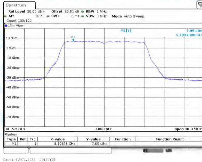
11A-BF_Ant4_5200
