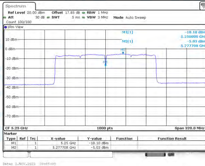
11AX160-CDD_Ant2_5250_UNII-2A
