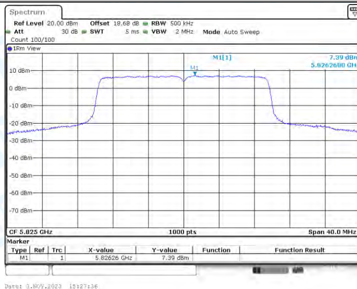
11AX20-CDD_Ant2_5825
