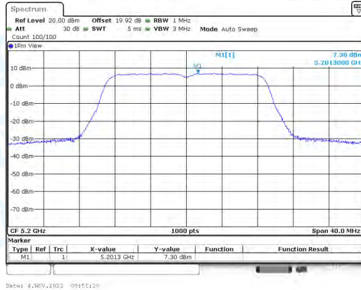
11N20-BF_Ant2_5200
