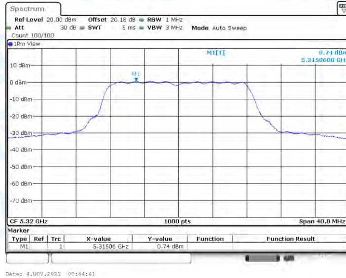
11A-BF_Ant3_5320
