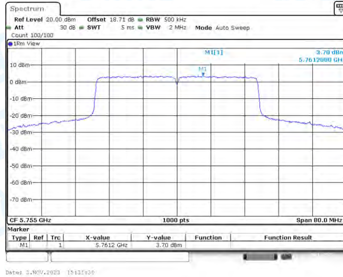
11AX40-CDD_Ant2_5755
