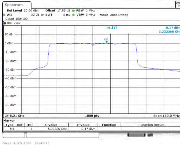
11AX80-CDD_Ant2_5210
