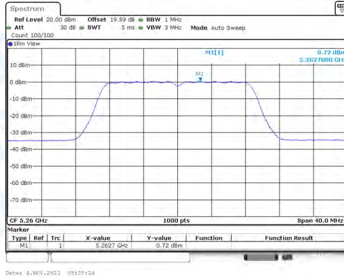
11N20-BF_Ant3_5260
