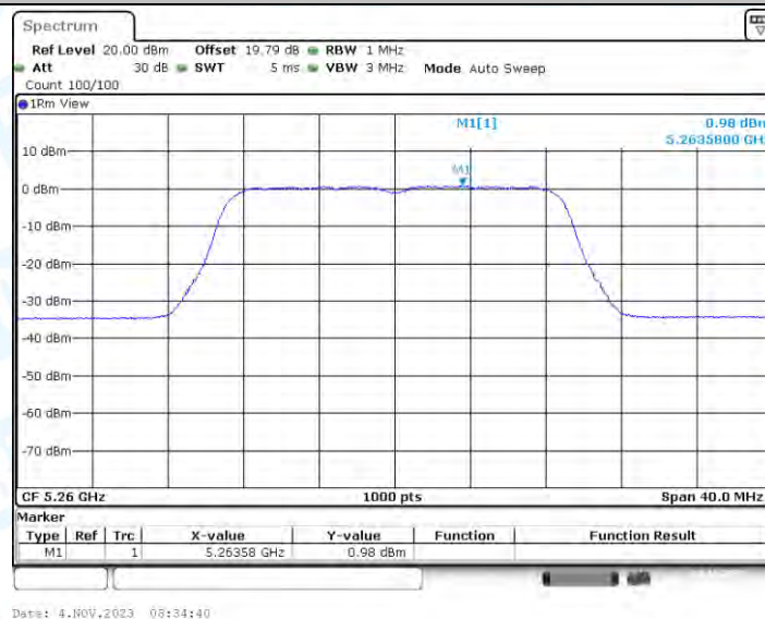
11N20-BF_Ant2_5260
