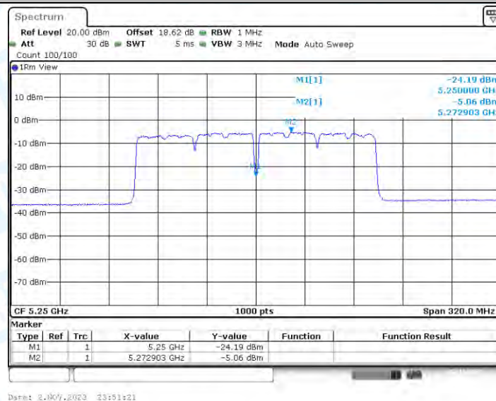
11AC160-CDD_Ant2_5250_UNII-2A
