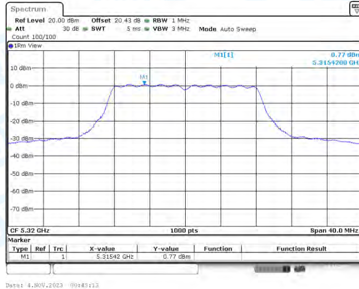
11A-BF_Ant4_5320
