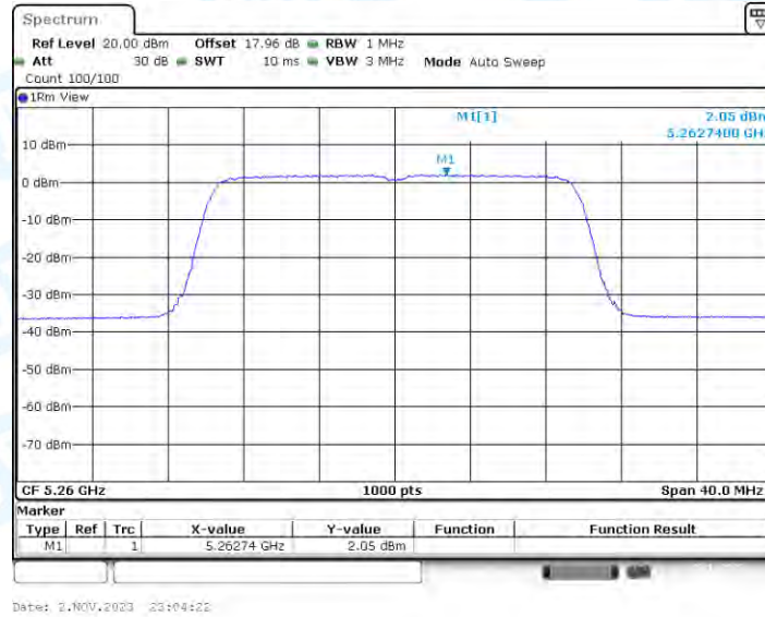
11AX20-CDD_Ant2_5260
