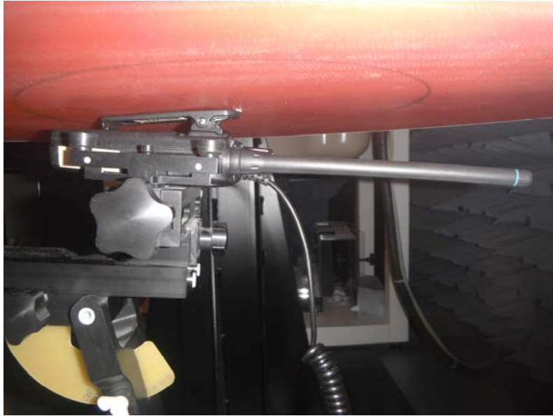
< FA-SC25V: 136MHz~150MHz; Blue Ring >
