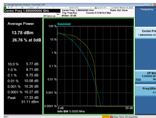
B2-1.4M-Mid CH-PAPR-QPSK
