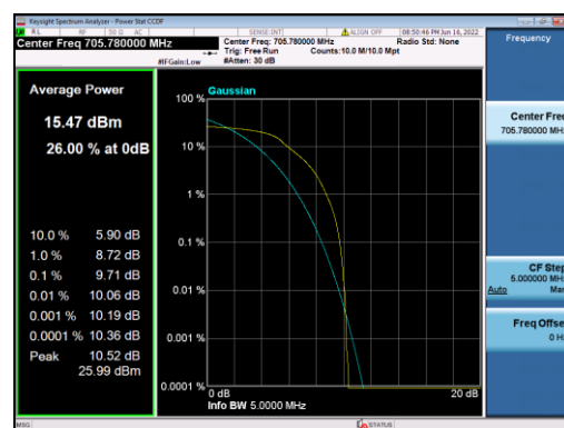
B12-5M-Mid CH-PAPR-QPSK
