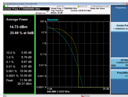
B4-5M-Mid CH-PAPR-QPSK
