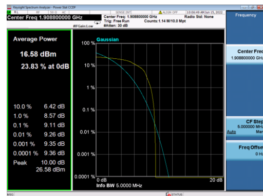
B2-10M-Low CH-PAPR-Q16
