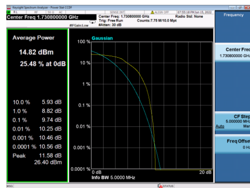
B4-5M-Mid CH-PAPR-Q16
