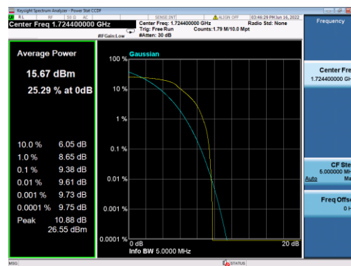
B4-20M-Mid CH-PAPR-QPSK
