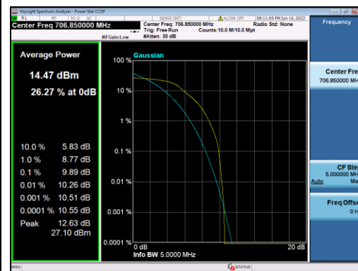
B12-3M-Mid CH-PAPR-QPSK
