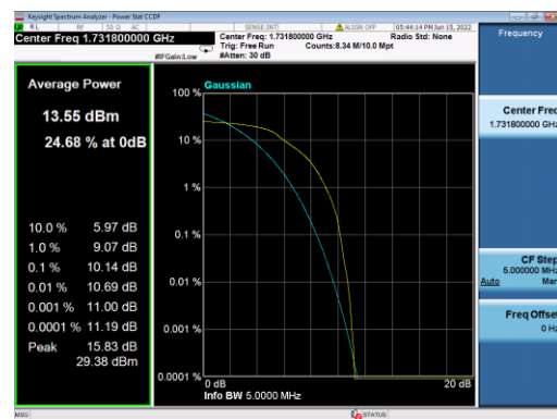
B4-3M-Mid CH-PAPR-Q16
