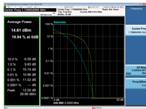
B4-10M-Mid CH-PAPR-Q16
