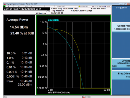
B2-5M-Mid CH-PAPR-Q16
