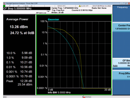
B2-3M-Mid CH-PAPR-QPSK
