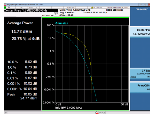
B2-5M-Mid CH-PAPR-QPSK
