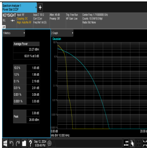
Band4-10MHz-QPSK-20000-1RB#0-PASS
