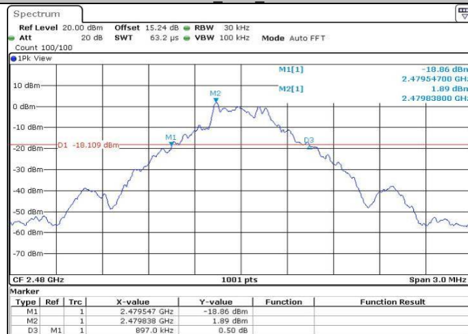
DH1_Ant1_2480
