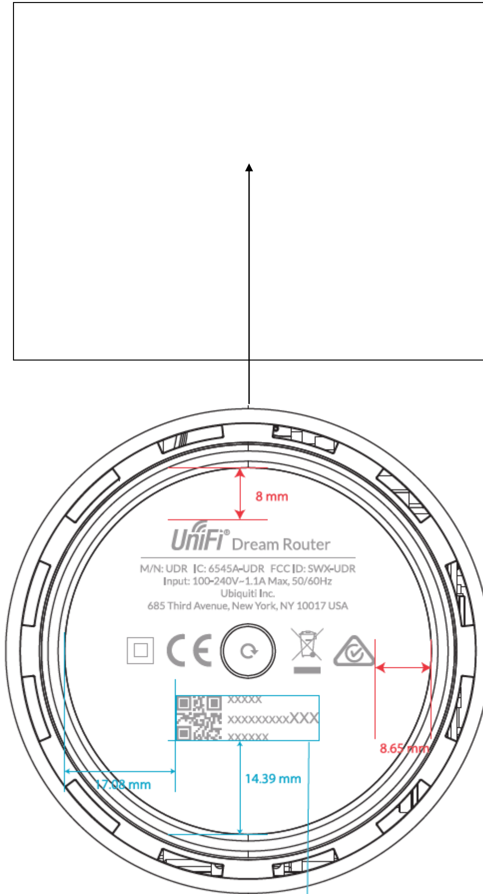
Bottom side
