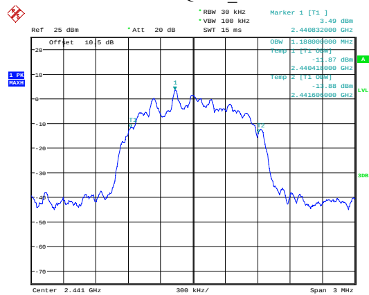
\pi/4 -DQPSK_Middle
