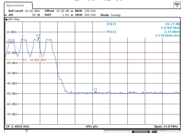
GFSK_Hopping_Upper
