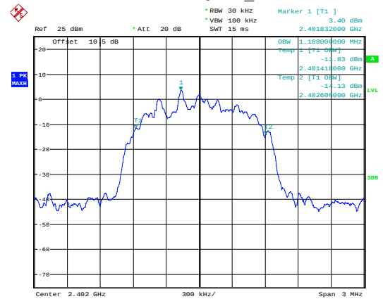
\pi/4 -DQPSK_Low
