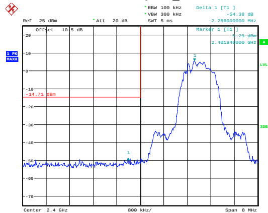
\pi/4 -DQPSK_Low
