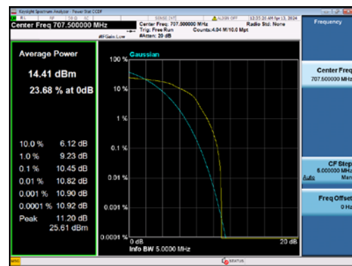
B12-1.4M-Mid CH-PAPR-Q16
