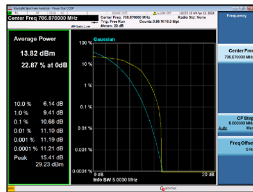
B12-3M-Mid CH-PAPR-Q16
