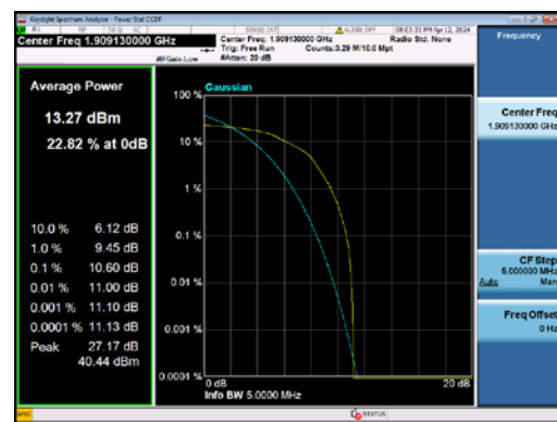
B2-3M-Low CH-PAPR-Q16
