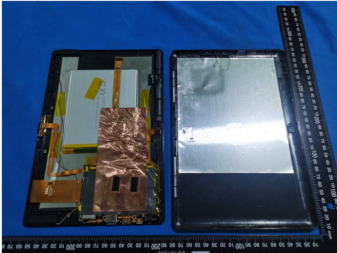
WIFI&BT&BLE Antenna
