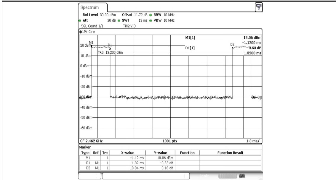
NTNV-802.11b-Ant2-2462
