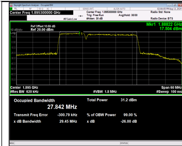
2-2-10MHz-20MHz-QPSK-QPSK-18956-19100-50RB#0-1 00RB#0-PASS
